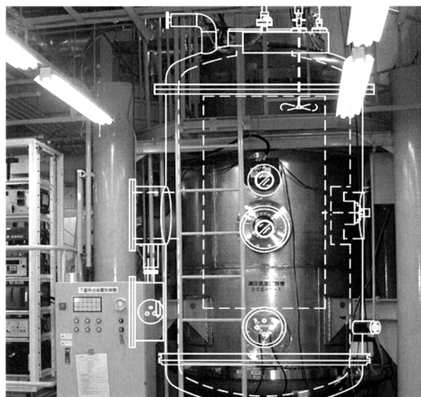
第3図 雲生成チェンバー. 気圧制御・断熱用の外チェンバーと温度制御用の内チェンバーから成る二重構造で、内チェンバー内が実験空間. 減圧による断熱冷却率に一致するように内チェンバーの壁温を制御し、実験空間内で断熱膨張 (雲生成) を再現する装置.
