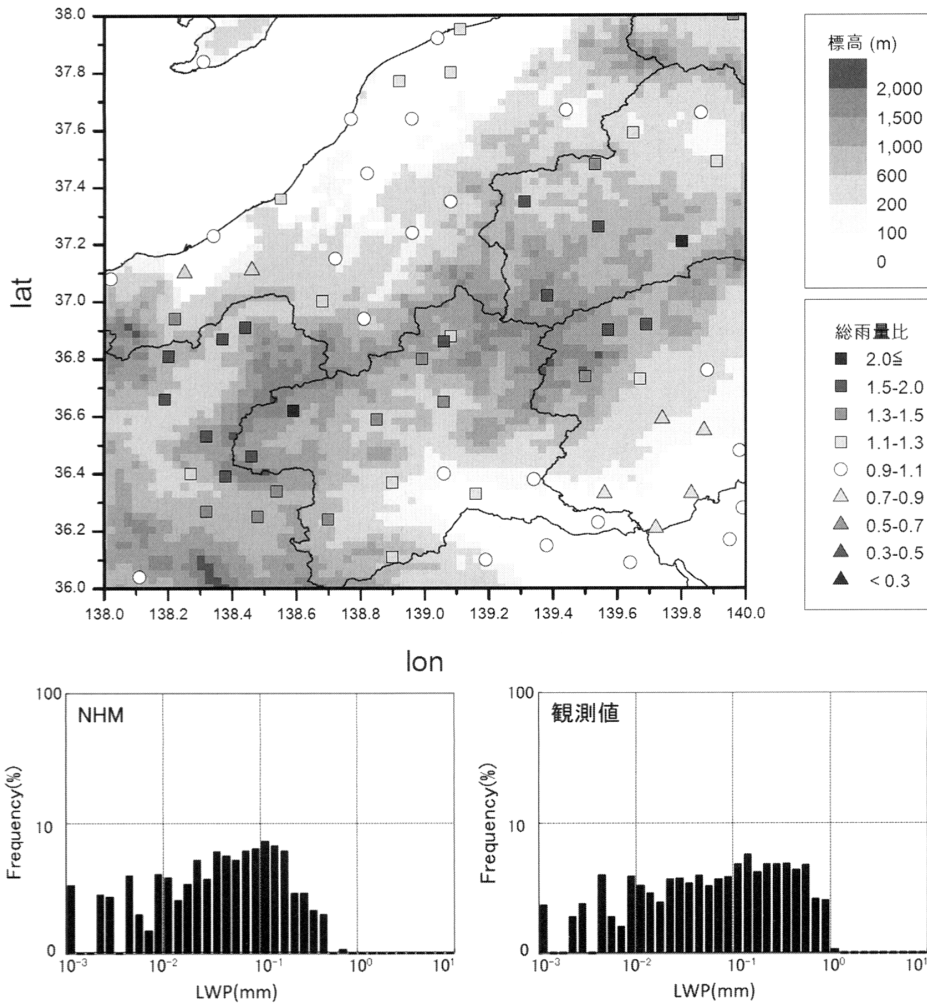
第8図 越後山脈周辺における1冬季間(2007年1月~2008年3月)の降水量の1 km-NHMによる計算値と固体降水粒子に対する雨量計の捕捉率を補正後の実測値の比(上段), 越後山脈風上側における1冬季間のLWP出現頻度の1 km-NHMによる計算値(左下図)とマイクロ波放射計による実測値(右下図). (小池ほか 2015)
