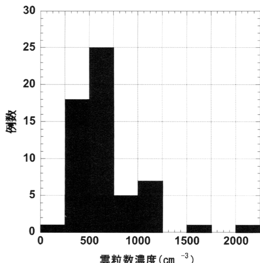
第1図 越後山脈上空における雲粒子濃度の出現頻度分布 (1997~2002年度冬季集中観測期間).
