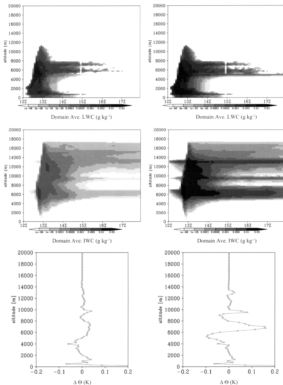
第6図 清浄大気中(左列)と汚染大気中(右列)に生成した積乱雲による領域平均液体雲・降水粒子(雲水+雨水)の混合比の時間高度断面(上段), 領域平均固体雲・降水粒子(雲水+雪+霰)の混合比の時間高度断面(中段), 及び6時間後の領域平均の温位偏差の鉛直分布(下段).
