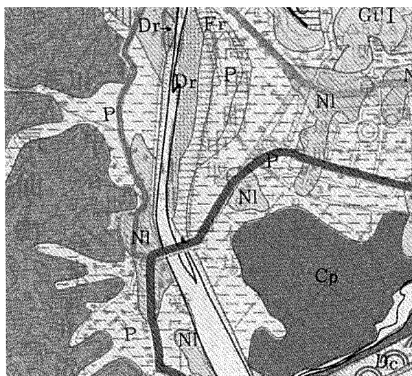
図1 地形分類図の例 岩手県(1975)より。主な記号の意味は、 P: 谷底平野および氾濫平野, NI: 自然 防, Dr: 浜および河原, Fr: 旧河道。
