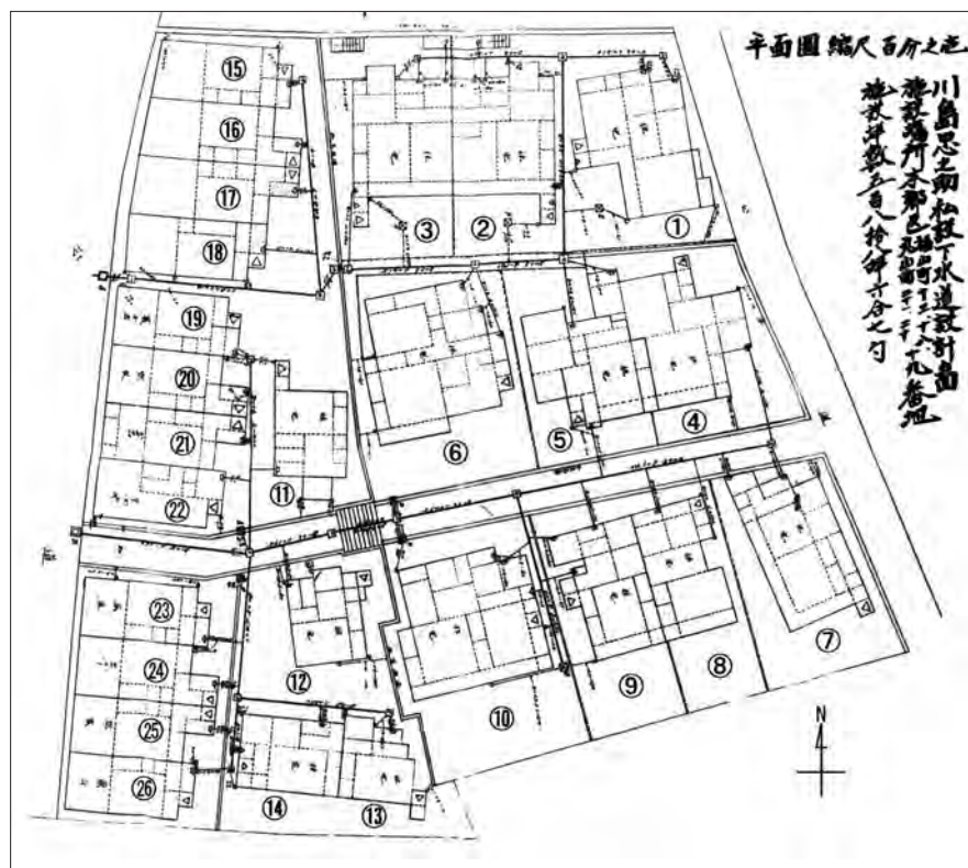
川島忠之助私設下水道設計図
