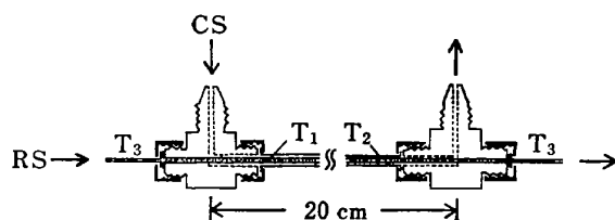
Fig. 2 Gas-diffusion unit
