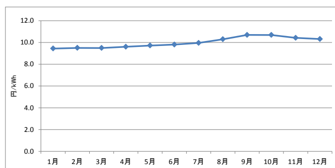
図 1-20 平均エネルギー購入単価：深夜電力
