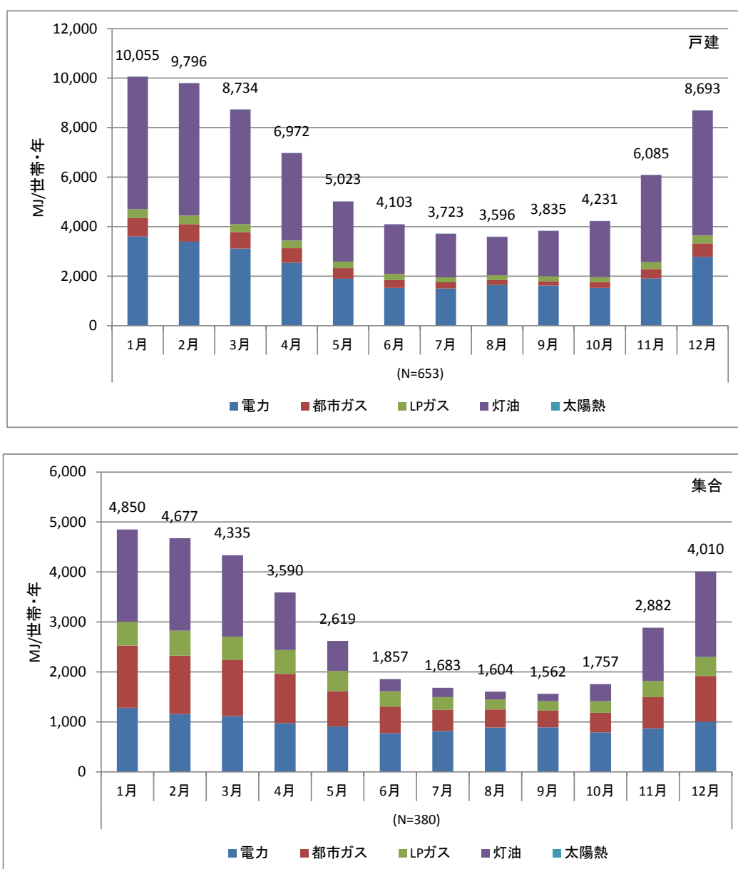
図 2-8 地域別エネルギー消費構造の月次変化（寒冷地）
