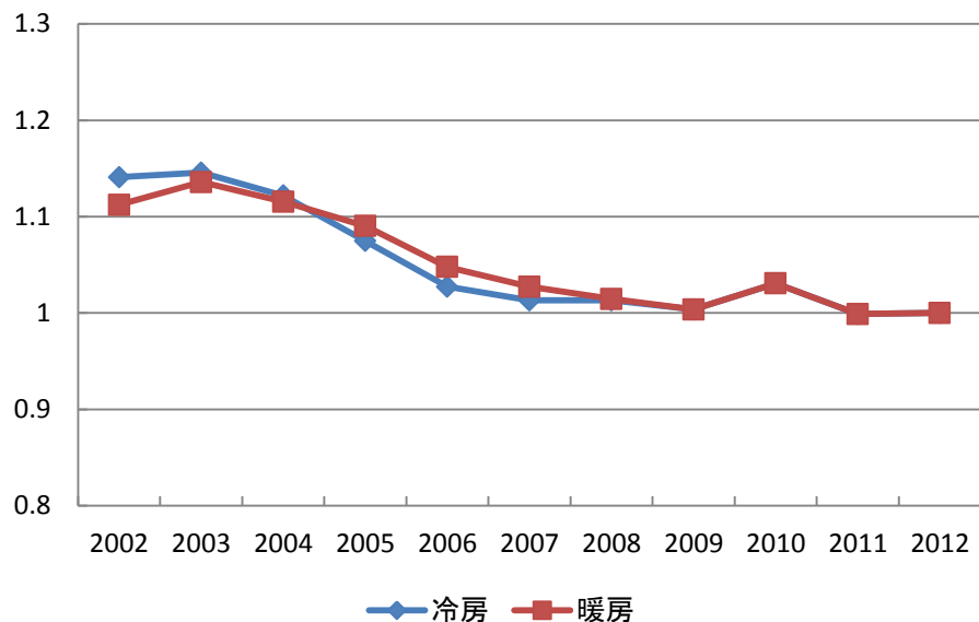
図 1-24 エアコンの期間消費電力量の推移 4
