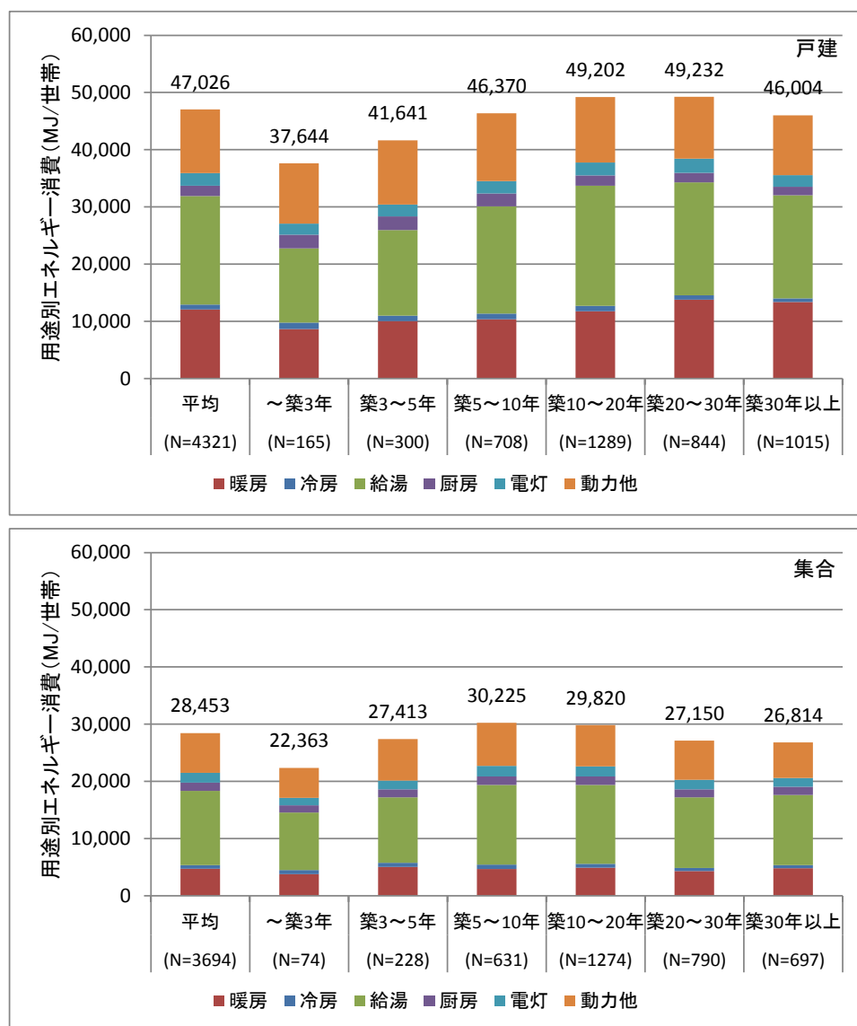
図 2-12 築年数別の用途別エネルギー消費原単位
