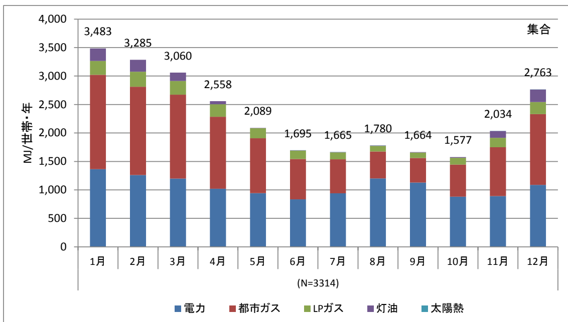
図 2-9 地域別エネルギー消費構造の月次変化（非寒冷地）
