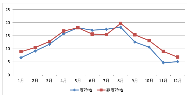
図 1-22 全天日射量の月別変化
