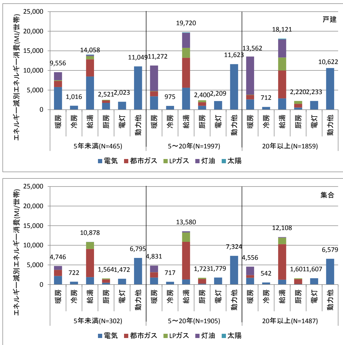
図 2-20 築年数別のエネルギー源別用途別エネルギー消費原単位
