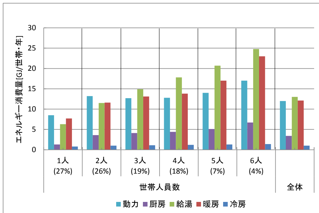
図 1-26 世帯人員別用途別エネルギー消費量（電中研試算結果）
