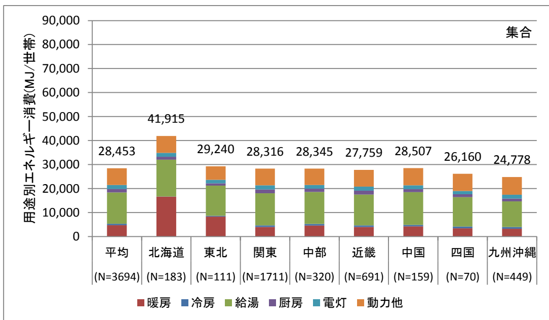
図 2-11 地域別の用途別エネルギー消費原単位
