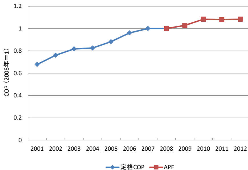
図 1-28 ヒートポンプ式給湯機の COP 推移 (2008 年=1 で規格化)
