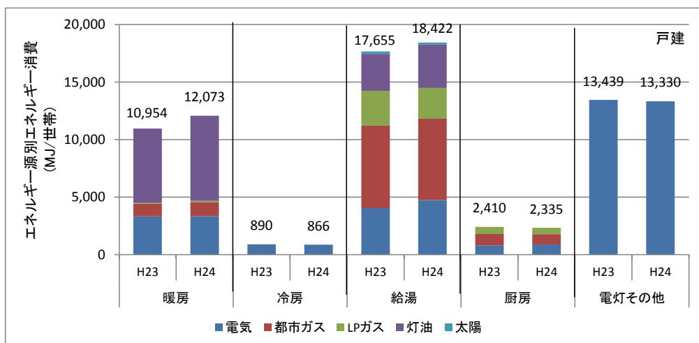
図 2-22 用途別のエネルギー消費原単位の経年比較（全国平均）
