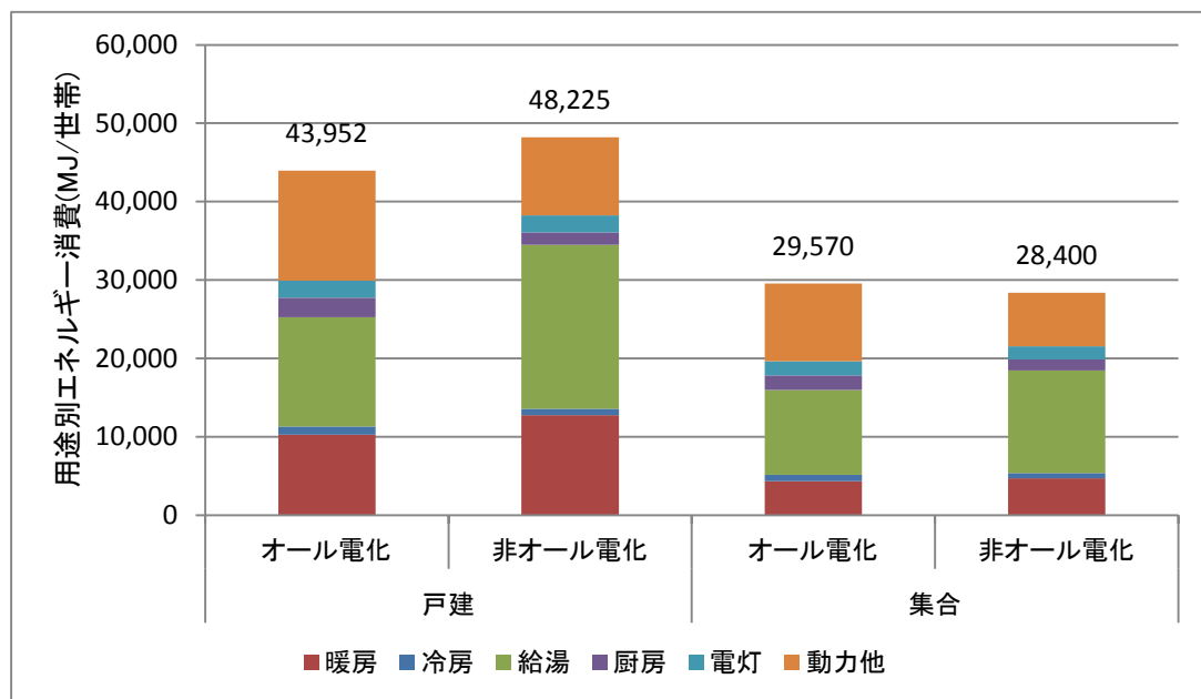
図 2-15 オール電化導入状況別の用途別エネルギー消費原単位
