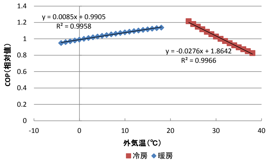
図 1-25 外気温別 COP（暖房-7℃のとき 1、冷房 31℃のとき 1 で規格化） （出典）「JIS 規格 C9612：ルームエアコンディショナの期間消費電力算出基準」より MRI 作成
