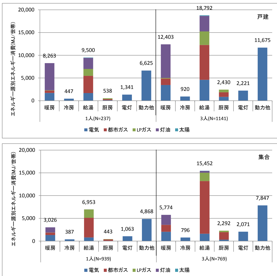
図 2-21 世帯人員別のエネルギー源別用途別エネルギー消費原単位
