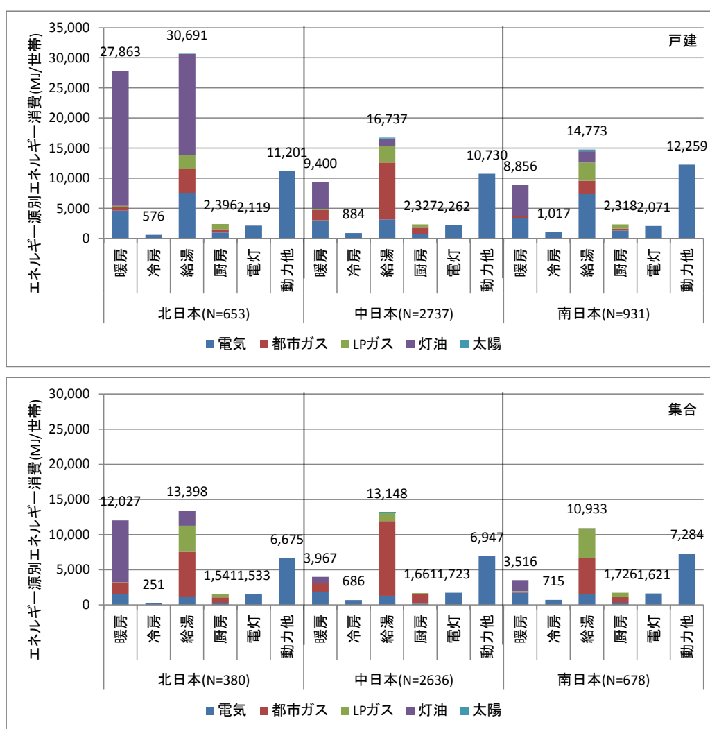
図 2-19 地域別のエネルギー源別用途別エネルギー消費原単位
