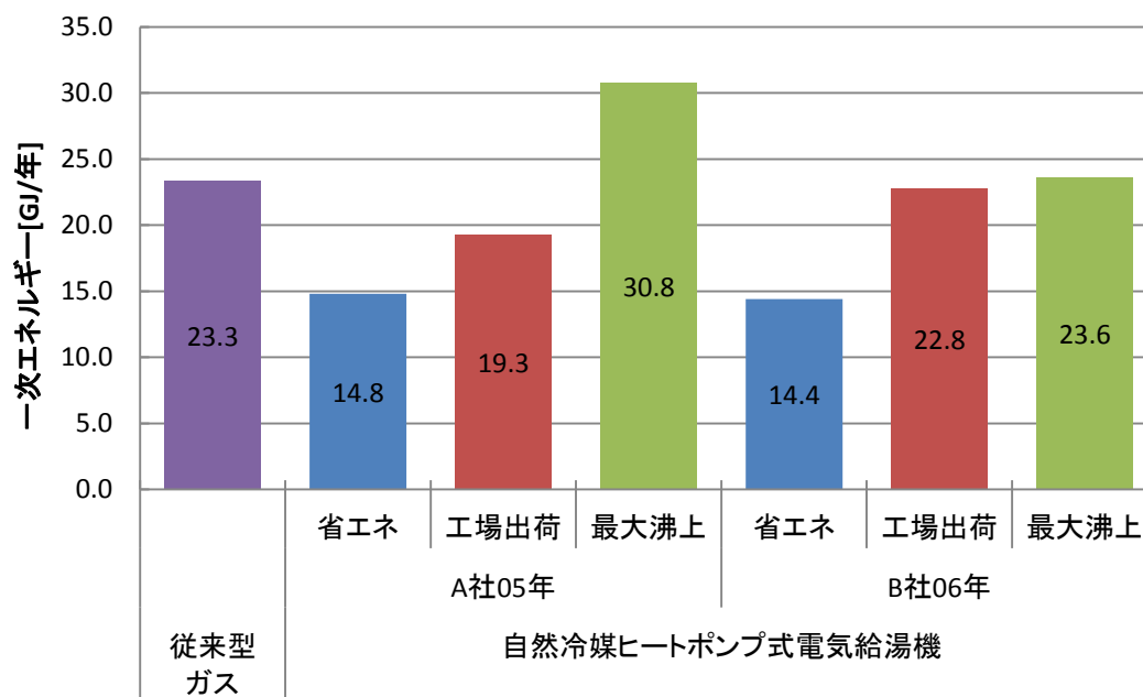
図 1-29 各種給湯機の一次消費エネルギー比較
