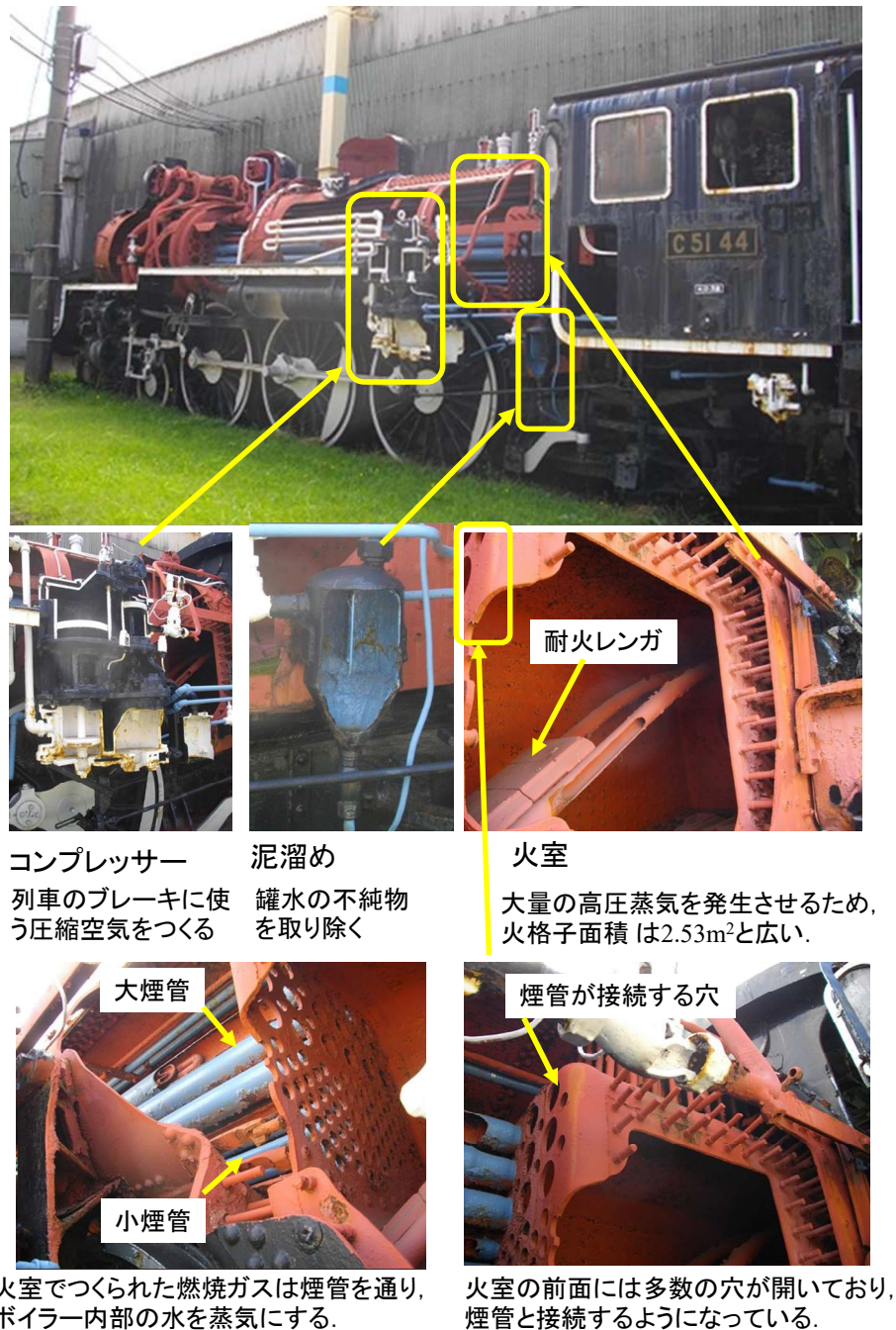
図2 C51-44号機関車の火室とその周辺
