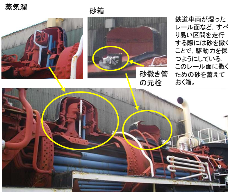
図3 ボイラーの上に設置されている蒸気溜と砂箱
