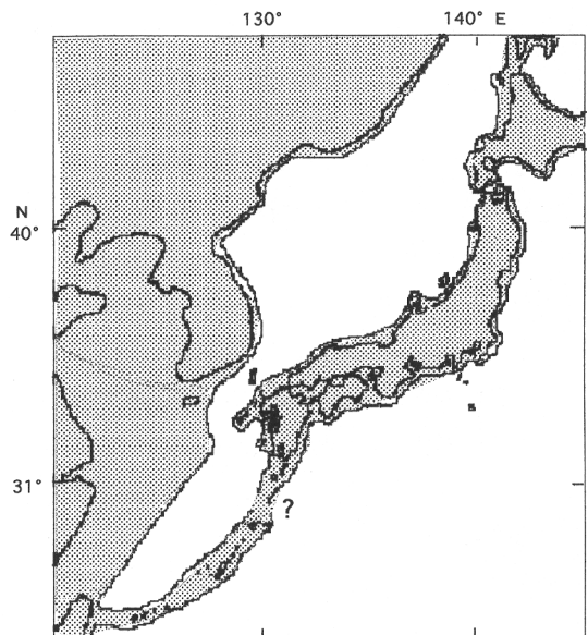
図-1 2～3万年前の日本の古地理図。アミ部が陸
