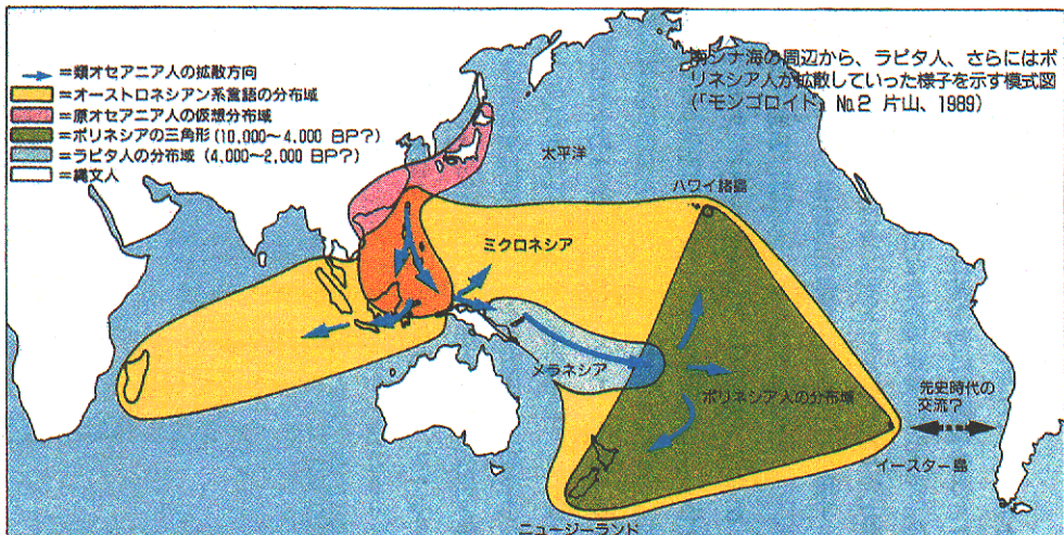
図-2 類オセアニア人の拡散を示す図（片山，1991による）
