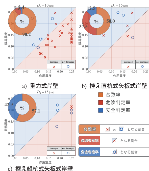
図-1 被災判定グラフによる被災検証結果
