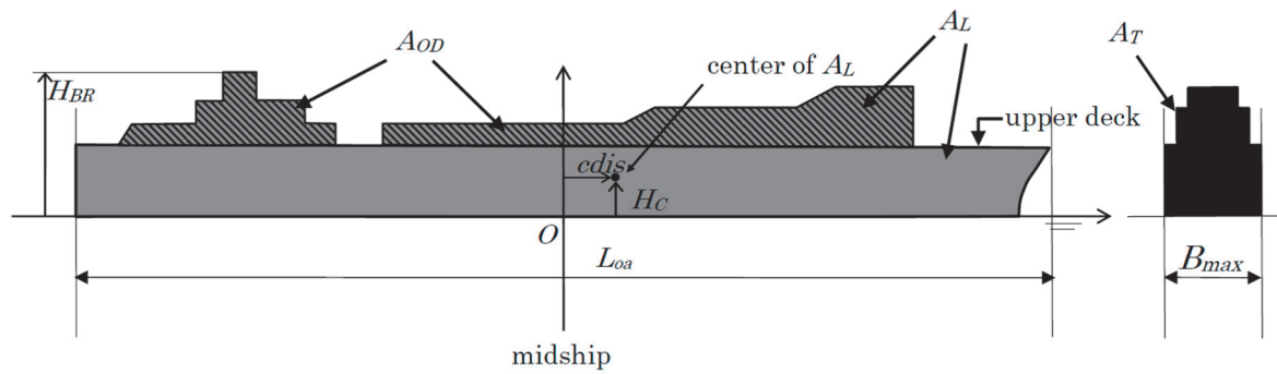
Fig. 12 Superstructure parameters
