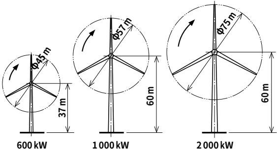
図8 大形風車の体格
