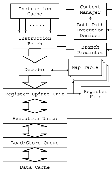
図2 両パス実行アーキテクチャの構成
