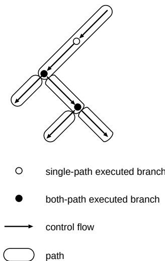
図3 パスの例
