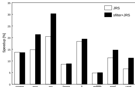
図7 分岐フィルタと両パス実行による性能向上率
