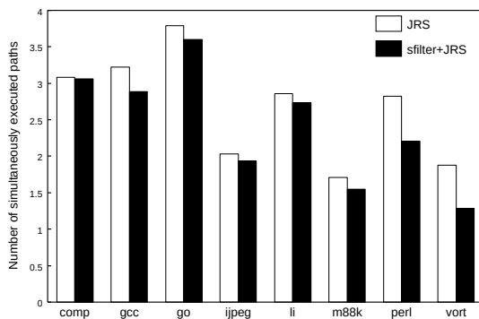
図10 同時実行された平均パス数 Fig. 10 Number of simultaneously executed paths.
