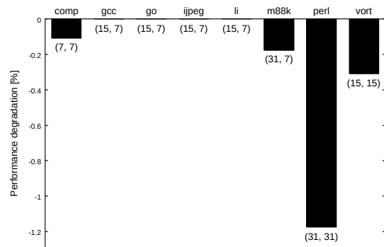
図8 ベンチマークごとの最適パラメータからの性能低下率
