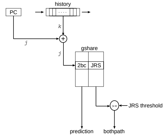
図 1 両パス実行判定機構の構成例
