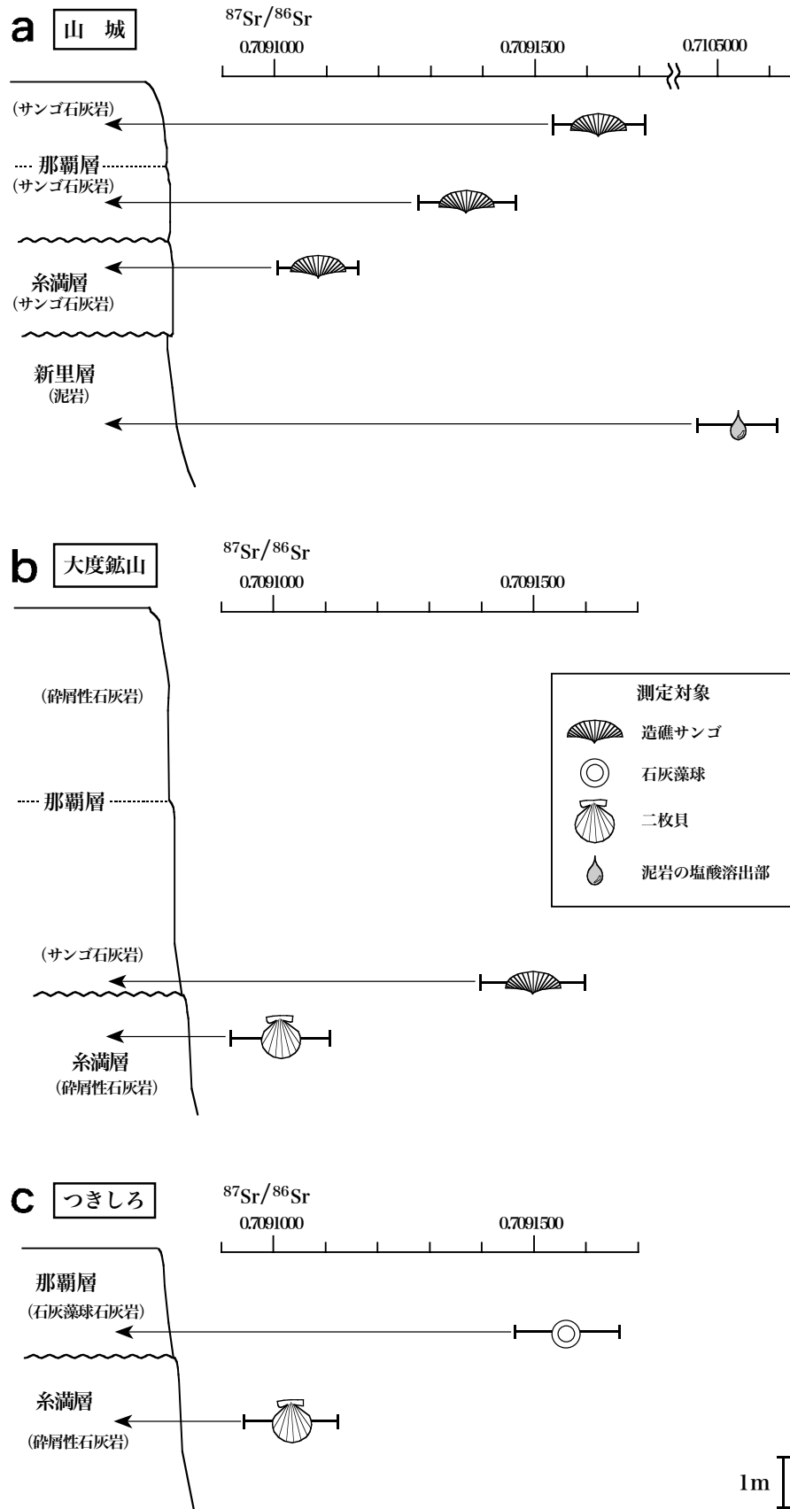
第7図 \text{Sr} 同位体組成測定地点の柱状図. a: 山城, b: 大渡鉦山, c: つきしろ.
