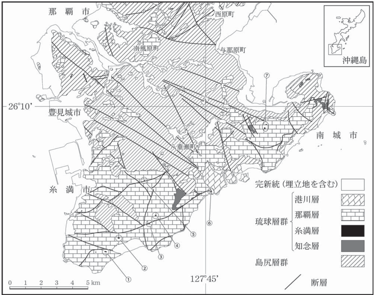
第1図 沖縄島南部地域の地質図及び地点図.
