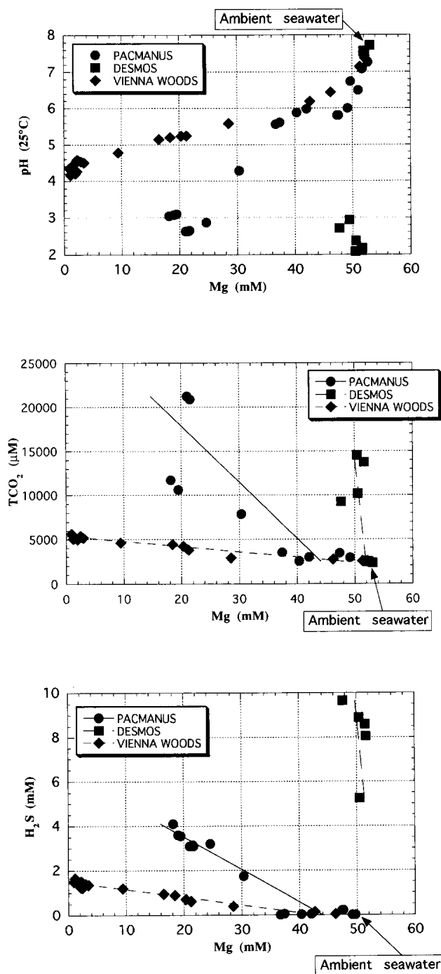
図2 マナス海盆の各熱水域から採取した熱水試料のMgに対するpH、全炭酸、硫化水素のプロット Fig. 2 Mg vs. pH, total carbonate and H 2 S relationships for the hydrothermal fluid samples taken from three hydrothermal sites in the Manus Basin.
