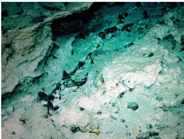
写真1 蛇紋岩海山山頂の割れ目に沿って密集する化学生物群集 Photo 1 Chemosynthetic animal community along the carbonate fissure.
