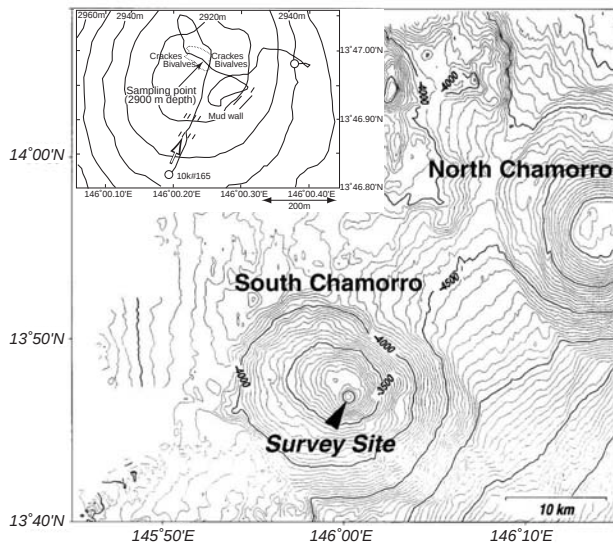
図1 チャモロ海山の海底地形と試料採集位置
