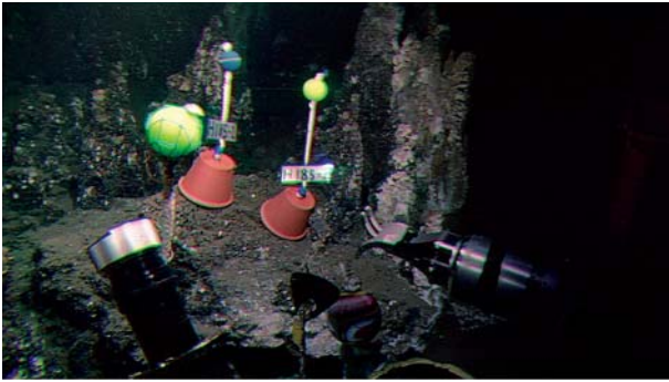
図2 明神海丘の Neoverruca sp.の優占する生物群集に設置されたマーカ―付き付着基盤。
