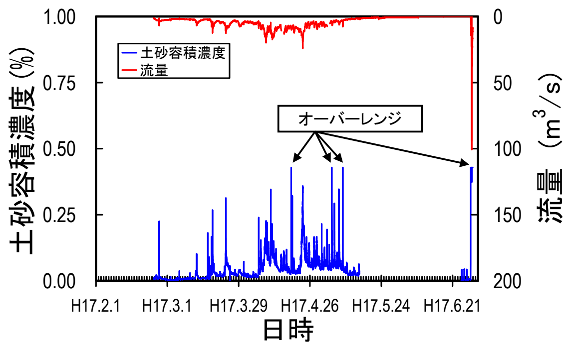
図－１２ 土砂容積濃度と流量の変化
