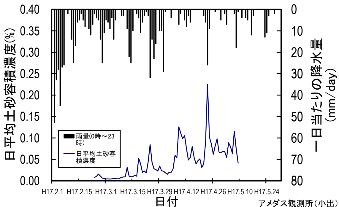
図－１８ 平均土砂容積濃度と降水量との関係
