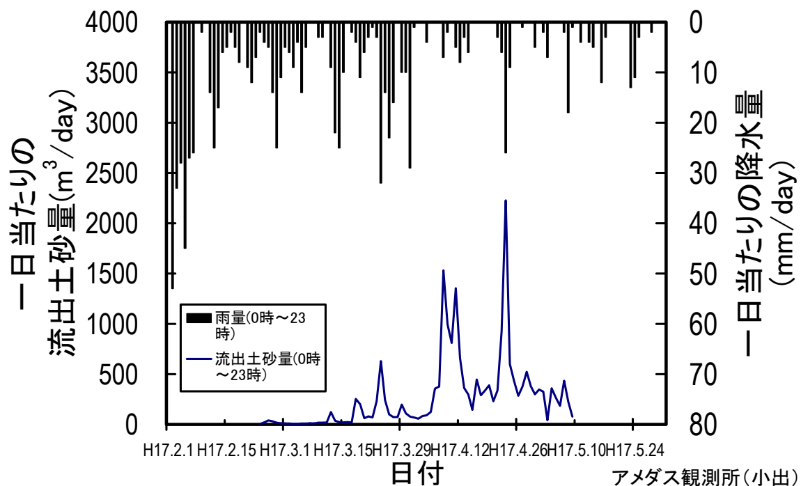
図－１６ 一日当たりの流出土砂量と降水量との関係
