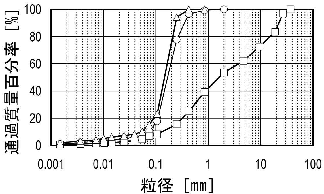
図一 4 小芋川大橋における河床材料の粒度分布 (平成 17 年 6 月 24 日採取)
