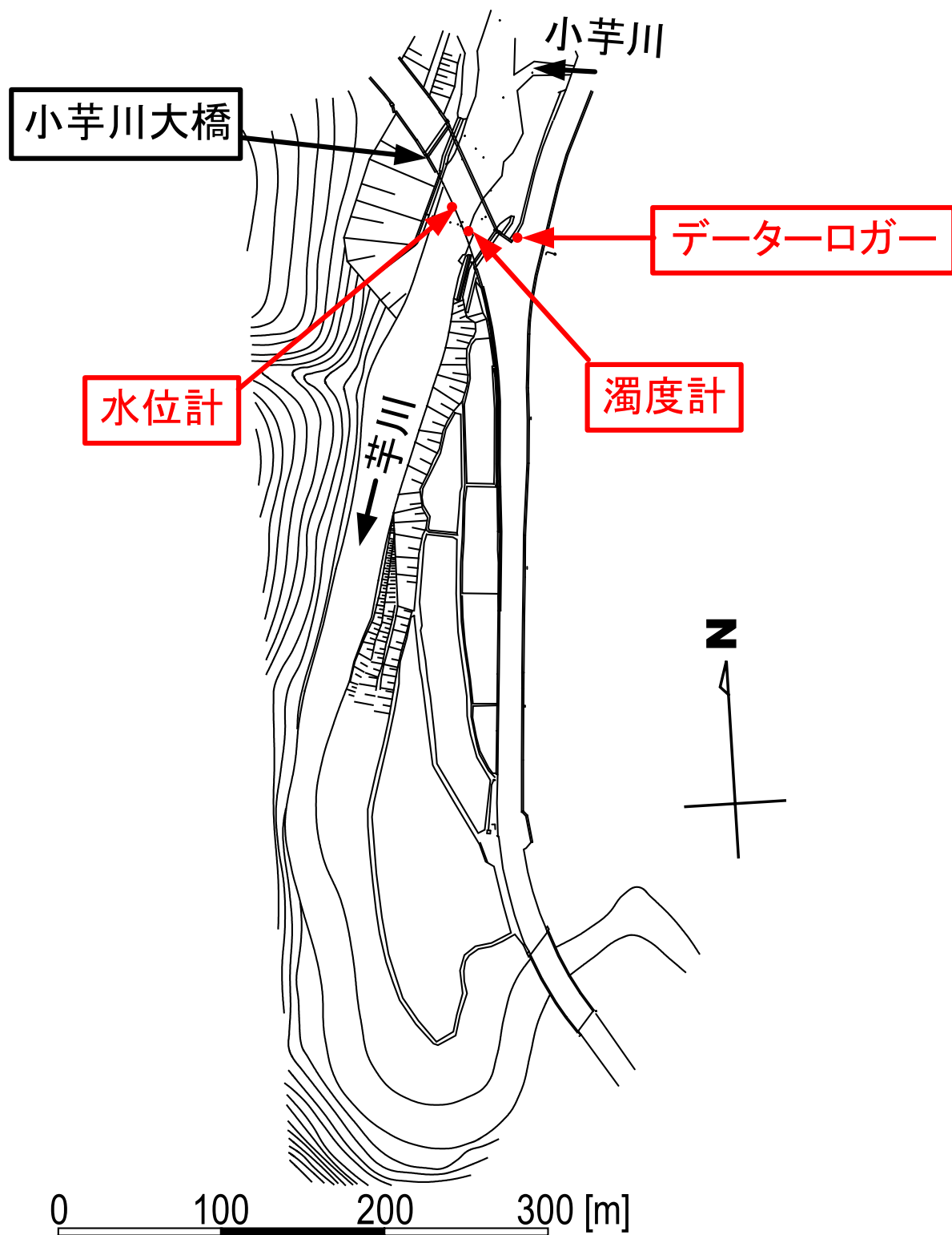
図－5 濁度計の設置箇所
