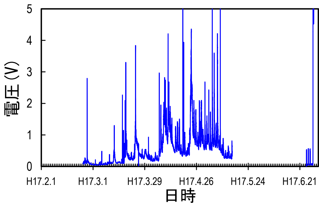
図－１１ 濁度の計測値の時間変化
