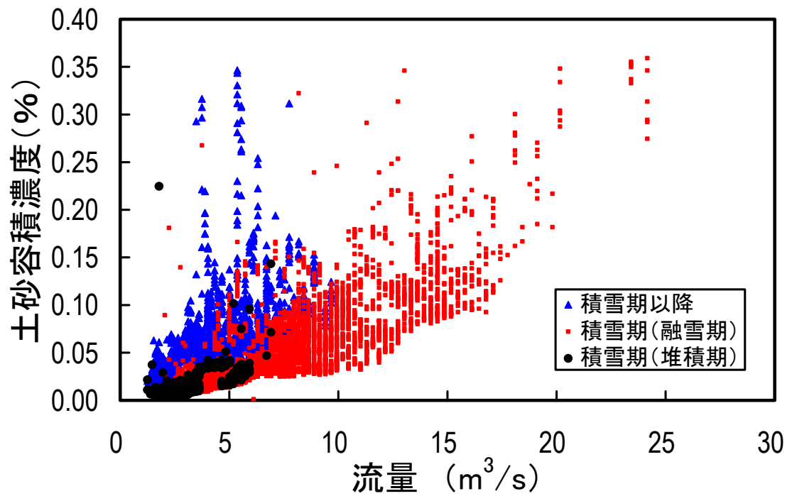
図－１３ 土砂容積濃度と流量の関係
