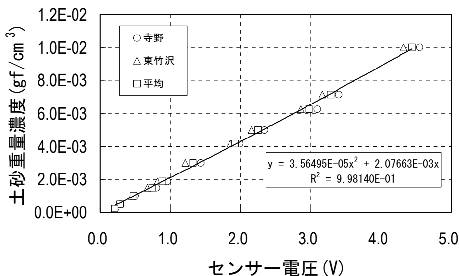
図-1.1 電圧 (V) - 土砂重量濃度 (gf/cm 3 ) の関係図
