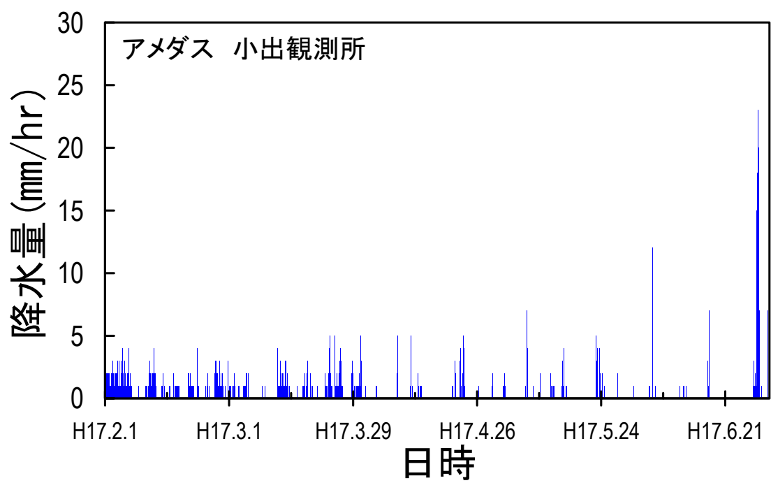
図－８ 降水量の変化
