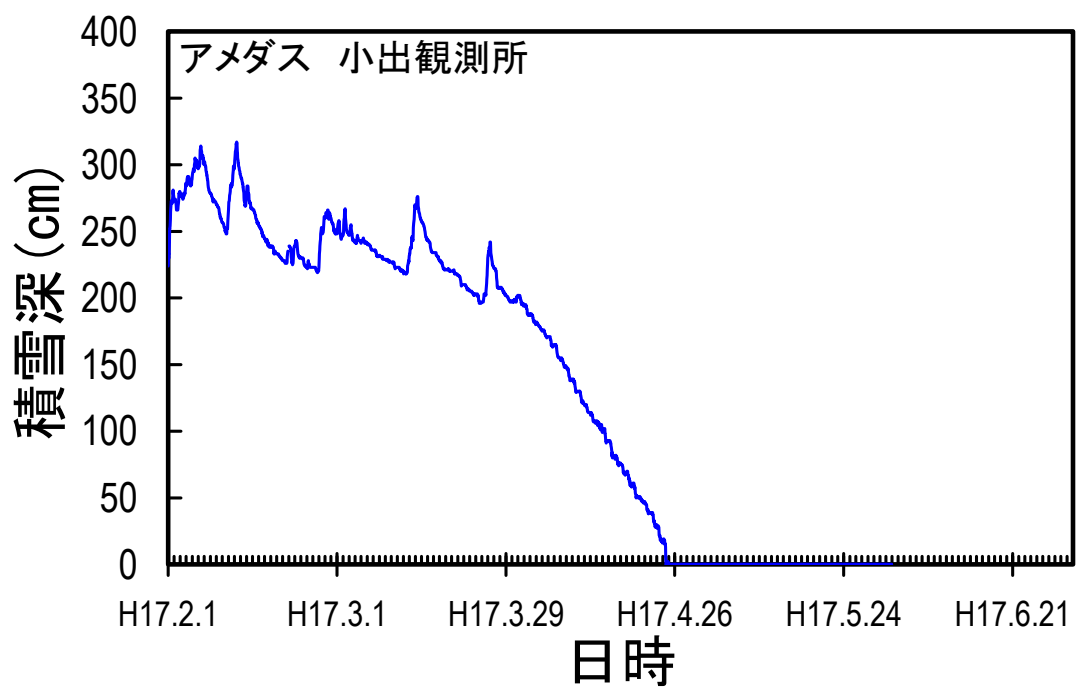
図－９ 積雪深の変化
