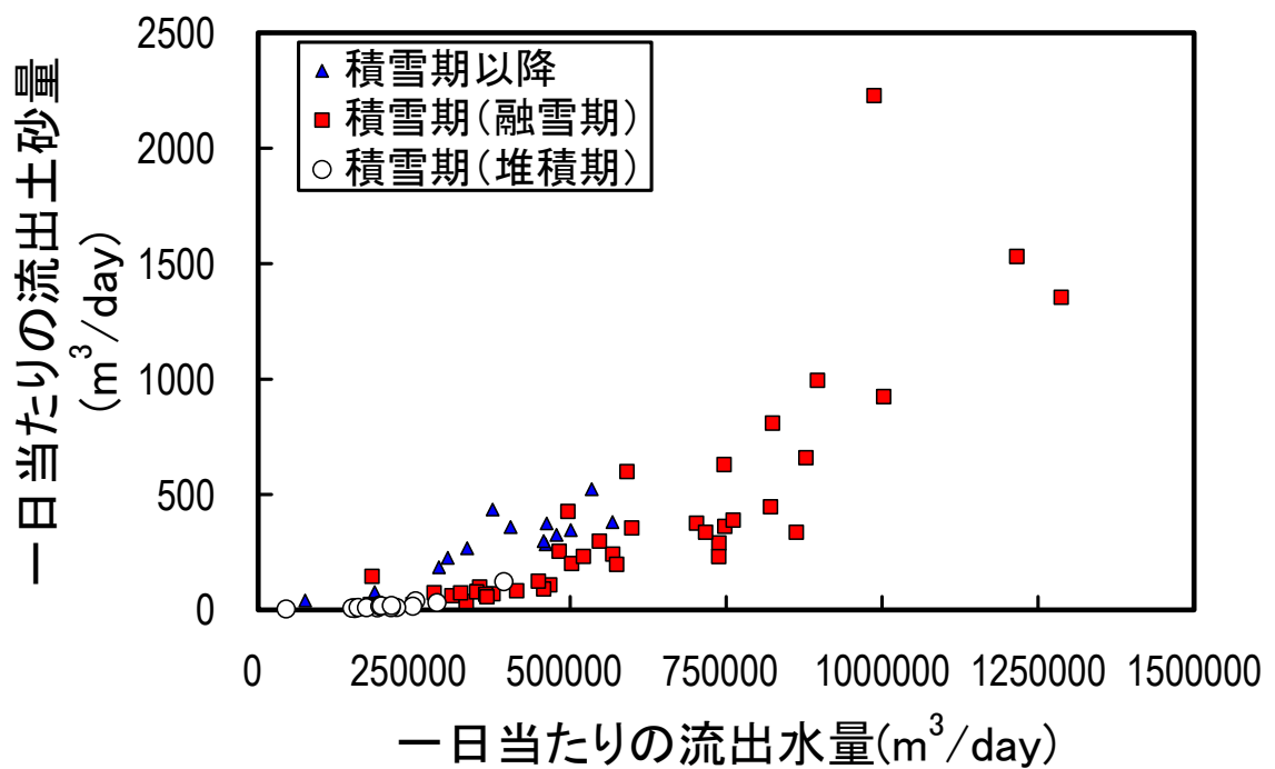
図－１４ 一日当たりの流出流量と流出土砂量の関係
