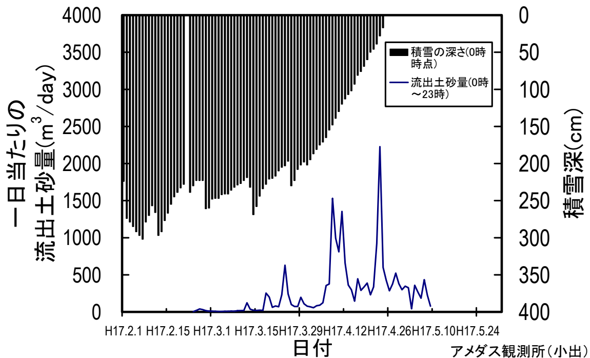
図－１５ 一日当たりの流出土砂量と積雪深との関係
