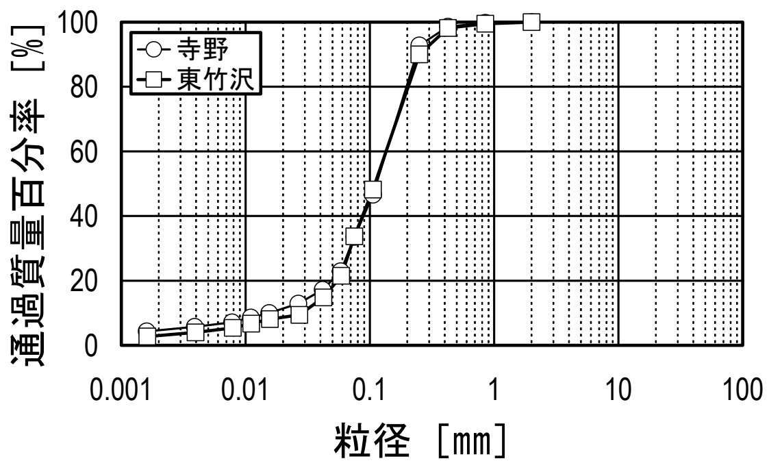
図一 3 河道閉塞を引き起こした土塊の粒度分布
