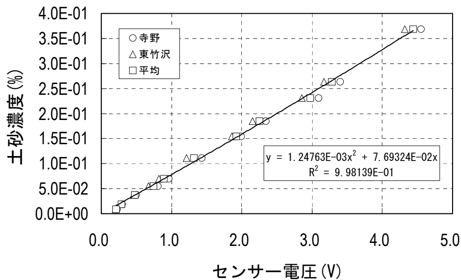
図-1.2 電圧 (V)－土砂容積濃度 (%) の関係図
