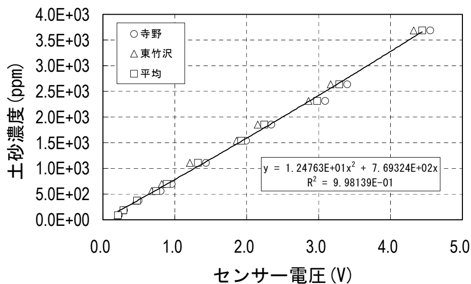
図-1.3 電圧－土砂濃度 (ppm) の関係図
