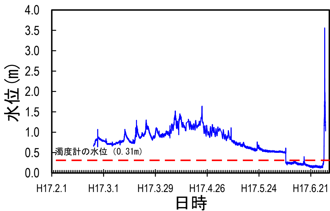
図－１０ 水位の時間変化
