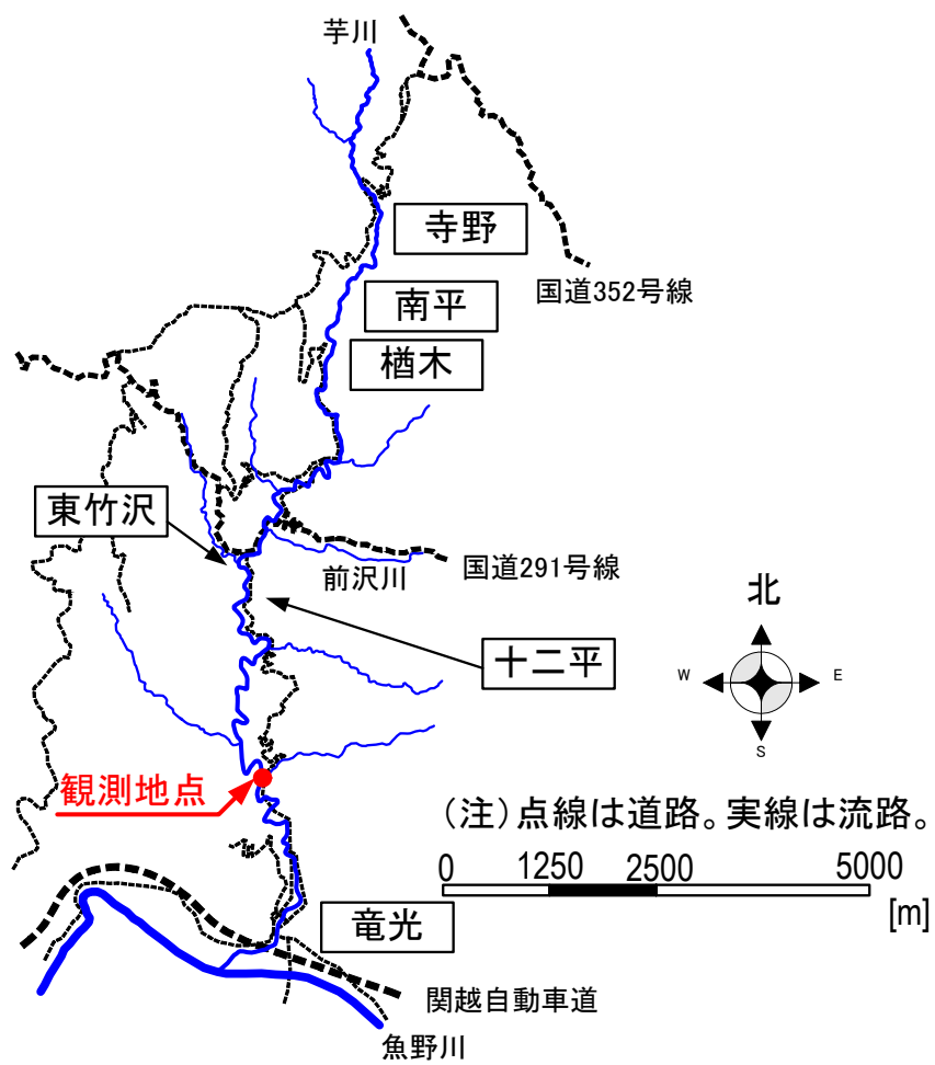
図－２ 芋川における主な河道閉塞発生箇所
