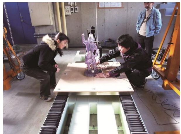
仏像縮小模型の振動台実験
