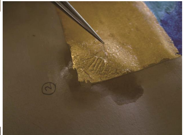
過去の修理に使用された ポリビニルアルコールの除去試験
