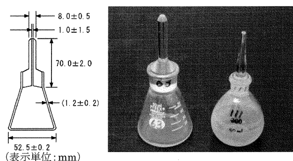
図－２ 用いた比重瓶（右側が従来のピクノメーター）
