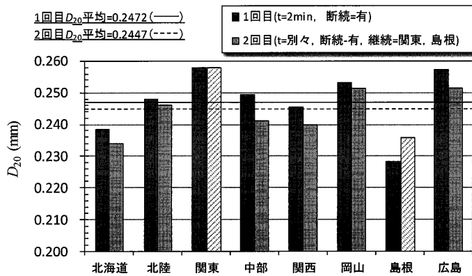
図—7 粒度（ふるい）試験における D_{20} の比較
