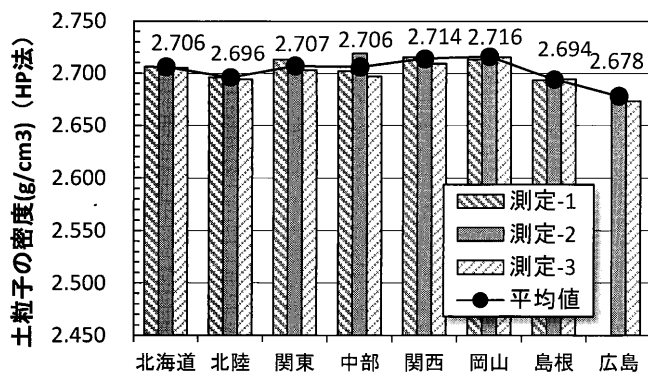
図—4 共通試料(藤森粘土)の土粒子の密度試験結果の比較(HP法)
