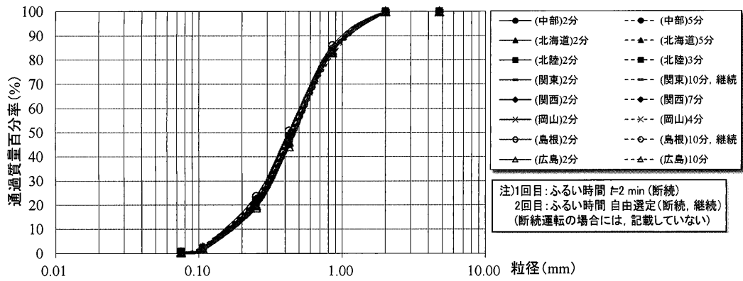
図—6 各組合による粒度（ふるい）試験結果
