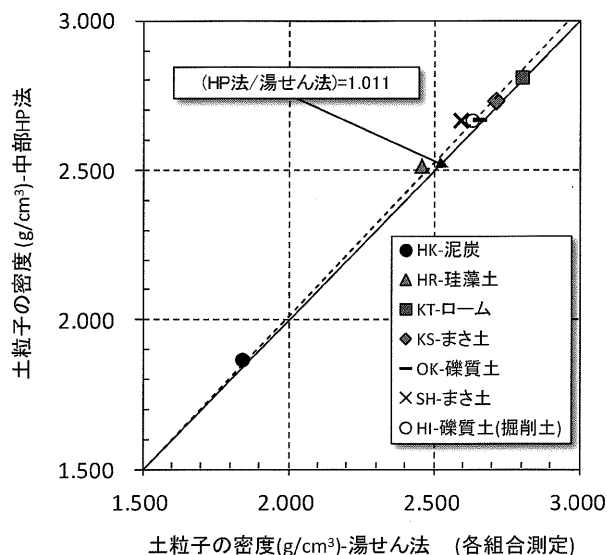
図－３ 湯せん法とホットプレート法の比較
