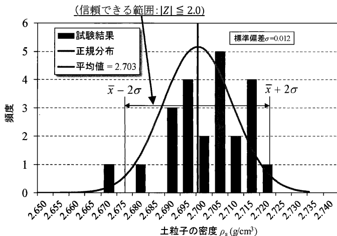
図—5 土粒子の密度のヒストグラム、正規分布曲線・信頼性範囲
