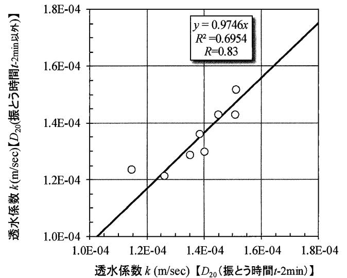
図—8 クレーガー式による透水係数の比較
