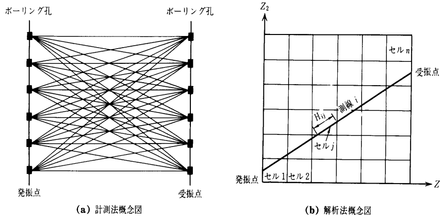
図—5.3 ジオトモグラフィーの概念
