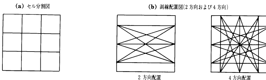
図—5.4 例題—5.3 (ジオトモグラフィー)
