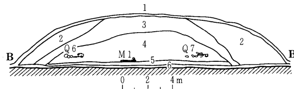
図-3 土墩墓断面図 (参考文献10)より引用)
