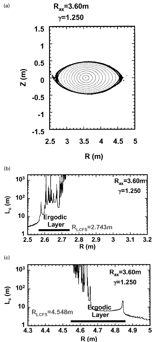
Fig. 3 LHD の横長断面位置における磁気軸位置が R_{ax}=3.6 m の磁場配位。ここでヘリカルコイルのピッチパラメータ \gamma は \gamma=1.25 である。閉じた磁気面がエルゴディック層で囲まれている。同図には、磁力線の接続長を主半径の関数としても示している[14]。
