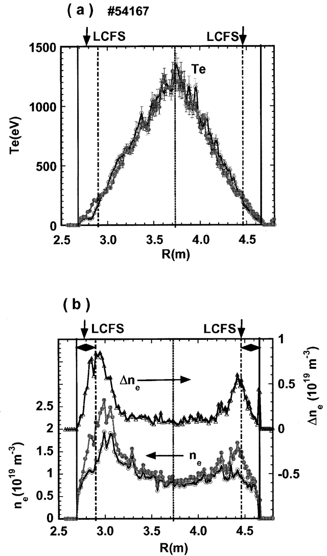
Fig. 7 R_{ax} = 3.6 m, \gamma = 1.22 , B_t = 0.75 T の条件で観測された LH 遷移の前後における電子温度(a)および電子密度(b)の径方向分布. 図(b)には、遷移に伴う電子密度の増分の径方向分布も示されている.
