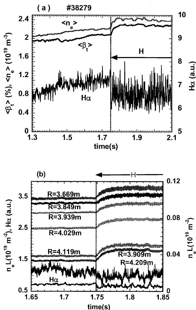
Fig. 4 (a)高ベータの水素プラズマにおいて観測された典型的な LH 遷移。ここで、磁場強度、磁気軸位置、ヘリカルコイルピッチパラメータおよび NBI 加熱の吸収電力はそれぞれ、 B_t = 0.75 T, R_{\text{ax}} = 3.55 m, \gamma = 1.254 および 4.3 MW である [9]。 (b) H \alpha 光およびレーザ干渉計の各種観測コード位置での信号の遷移前後における詳細な時間変化。ただし、 R = 4.209 m での干渉計信号は右側のスケールとする。
