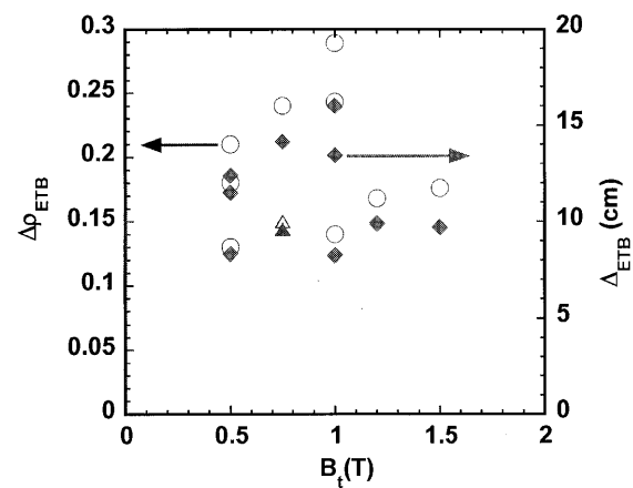
Fig. 8 ETB 幅のトロイダル磁場強度に対する依存性. 中実および白抜き記号は、それぞれ ETB 幅 \Delta_{ETB} およびプラズマ平均小半径で規格化した ETB 幅 \Delta\rho_{ETB} を意味している. 三角および円の記号は、それぞれ電子温度分布および電子密度分布から評価された ETB 幅を示している.
