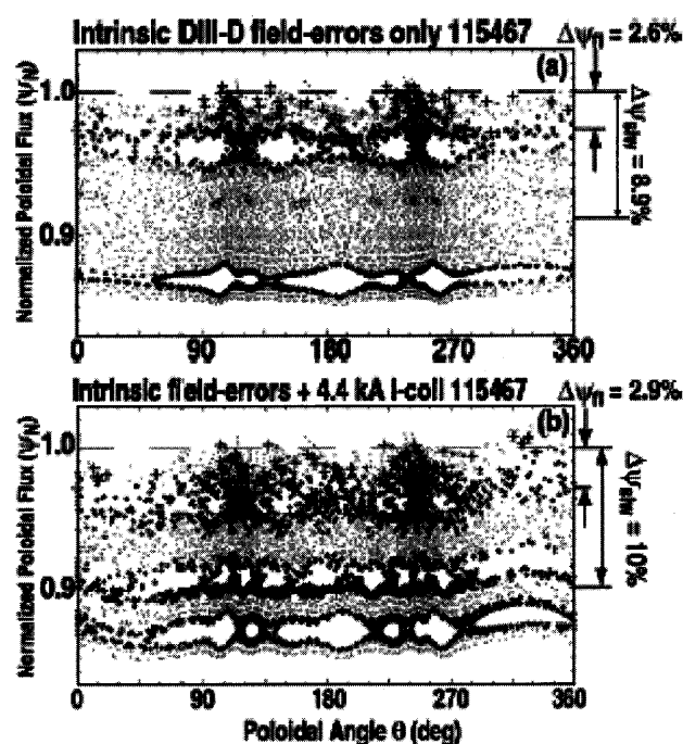
Fig. 2 (a)実測した誤差磁場を考慮したときの DIII-D の周辺磁場のポアンカレプロット。(b)誤差磁場に加え 4.4 kA の電流を I コイルに流し n=3 の磁場摂動を印加したときの DIII-D の周辺磁場のポアンカレプロット[13]。最外殻磁気面より内側の“+”印をつけた磁力線はセパトリックス外につながっており、最終的には炉壁に至っている。
