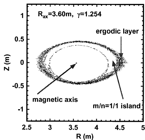
Fig. 9 LHD において LID 磁場の印加により m/n = 1/1 磁気島幅を増大させたときの周辺磁場のポアンカレプロット[15]。
