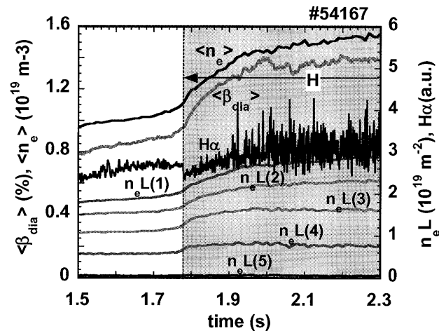
Fig. 5 磁気軸位置 R_{\text{ax}} = 3.6 m, \gamma = 1.22 の磁場配位において B_t = 0.75 T のときに観測された中程度のベータ値のプラズマで観測された LH 遷移 [15]。
