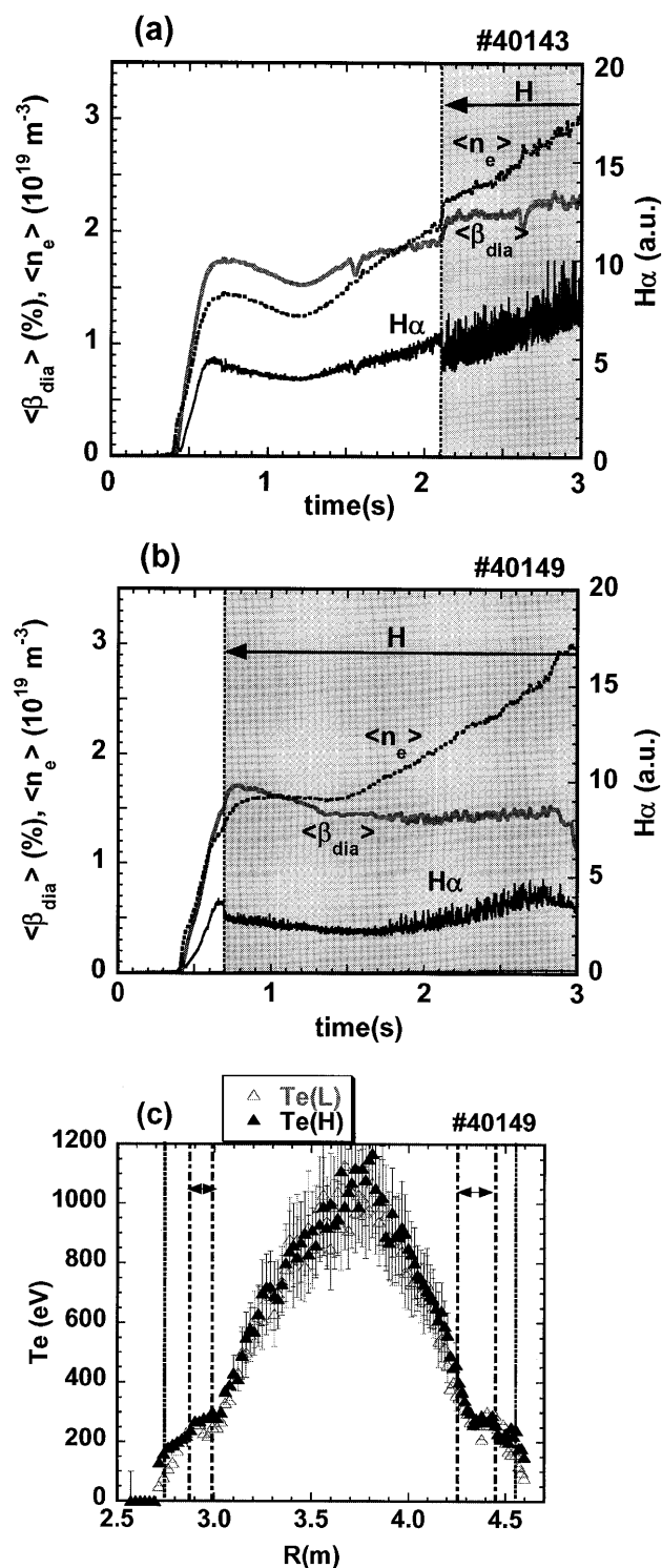
Fig. 10 (a)小さな LID 磁場印加により m/n = 1/1 磁気島を消去したときの ETB プラズマにおける平均電子密度、反磁性計測による平均プラズマベータ値および H \alpha 光の時間変化。(b)大きな LID 磁場印加により m/n = 1/1 磁気島を拡大したときの ETB プラズマの時間的振る舞い。(c)図(b)に示したショットでの LH 遷移の直前 ( t = 0.669 s) と直後 ( t = 0.769 s) の電子温度の径方向分布。点線の垂直線は、真空磁場における最外殻磁気面の位置を示している。また、2本の一点鎖線の間に示した水平の矢印は、真空磁場中に発生させた m/n = 1/1 磁気島の幅を示している[15]。
