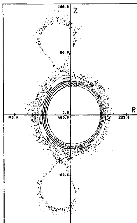
Fig. 1 ASDEX トカマク装置において、ポロイダル磁場コイルの設置誤差が数 mm あるとしたときの周辺磁場のポアンカレプロット。このような誤差磁場によりポロイダルダイバータのセパトリックスのすぐ内側に磁気島とエルゴディック層が形成される[12]。
