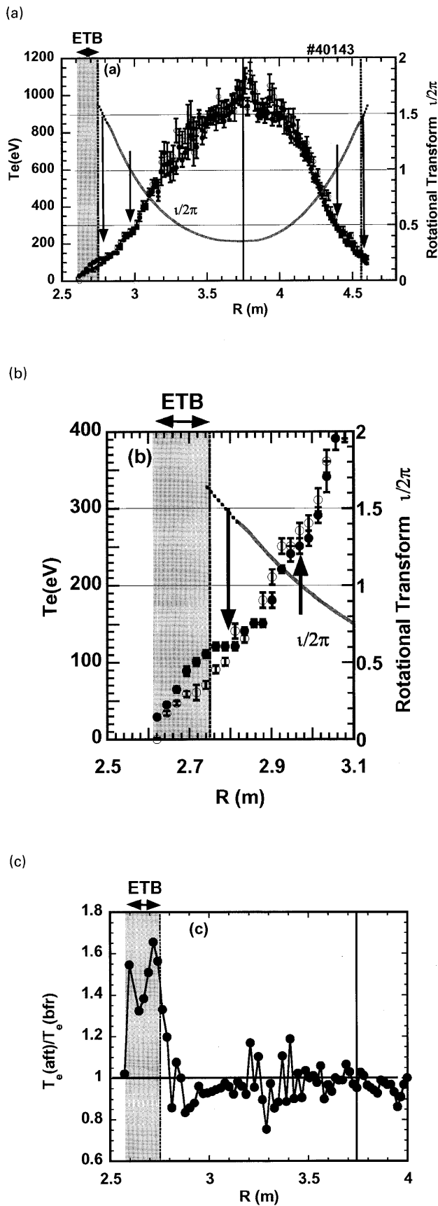
Fig. 6 (a) R_{ax} = 3.6 m, \gamma = 1.254 , B_t = 0.75 T の条件で観測された LH 遷移の前後の電子温度の径方向分布の比較[9]. (b)(a) に示した分布の周辺部の拡大図. (c) 遷移に伴う電子温度の増分の径方向分布.
