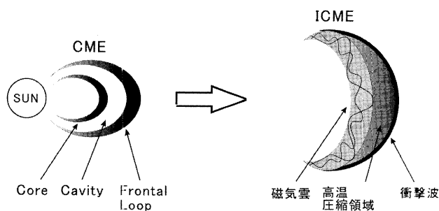
図4 コロナと惑星間空間における CME 構造の模式図。
