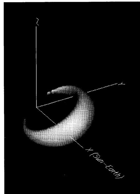
図9 シンチレーション観測から求められた2000年7月14日のCMEイベントの3次元構造。XY面は黄道面で、X軸は太陽-地球方向。原点は太陽の位置で、各軸の長さは1AU。([9]より転載)
