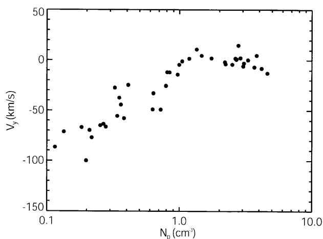
図7 太陽自転方向の太陽風速度と密度との相関図。([4]より転載)
