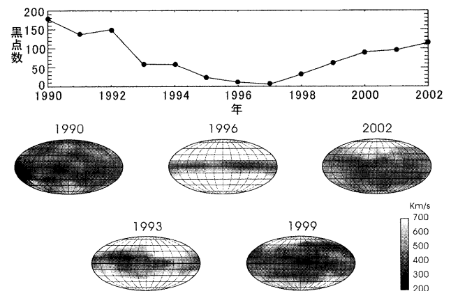
図2 太陽速度緯度経度分布の太陽黒点活動依存。速度分布はIPS トモグラフィー解析で得られた。
