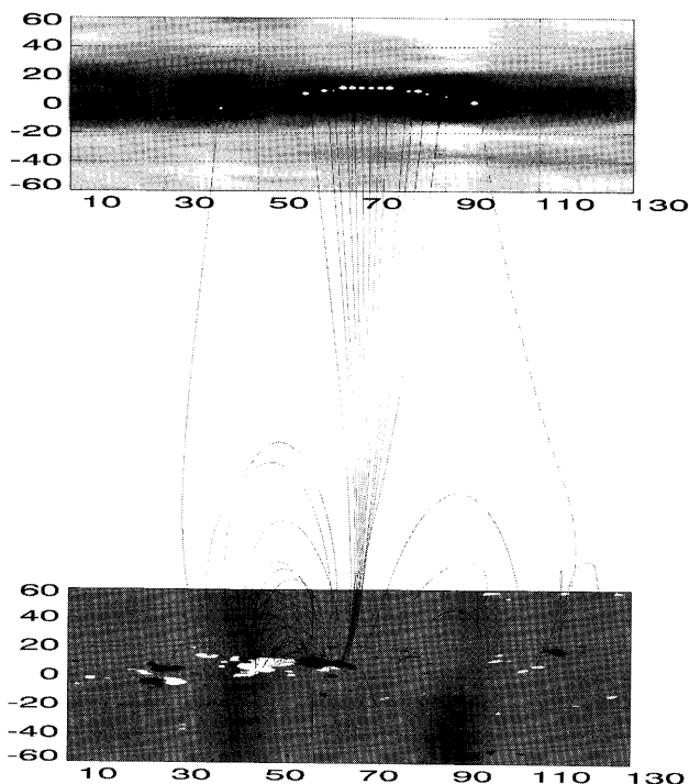
図8 太陽活動極小期に現れた低速ストリーマー。上図は、2.5 太陽半径の距離にプロットした太陽風速度の緯度経度分布図。経度70度付近の黒色の領域は速度370 km/s 以下を表す。下図は、米国キットピーク観測所で観測された太陽面上の磁場分布で、黒白で極性を表している。上図と下図を結ぶ細線は、ポテンシャル磁場で、太陽風の流管を表す。([3]より転載)
