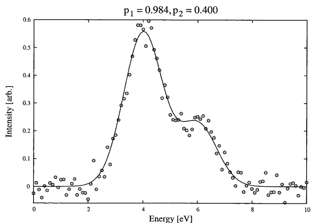
図4 近接する2つのガウシアンピークの和。
