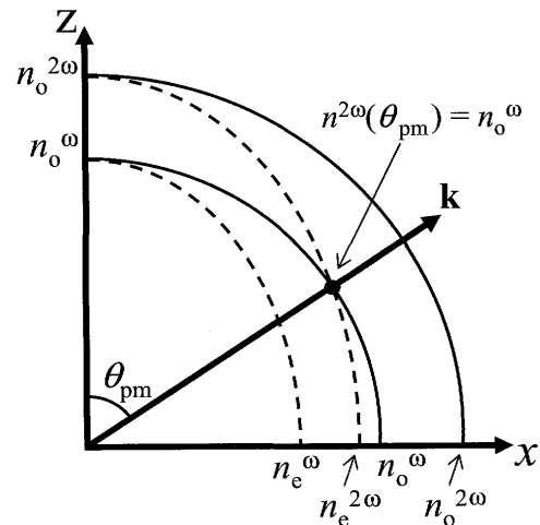
図2 負の一軸性結晶の第2高調波発生（タイプ1）の位相整合時の屈折率の関係．位相整合角 \theta_{\text{pm}} の時に n^{2\omega}(\theta) = n_o^\omega となる．
