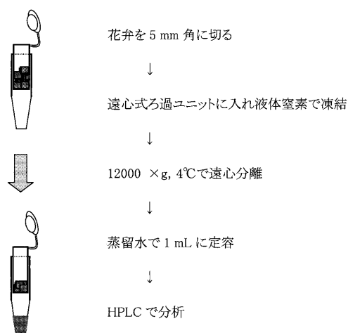
第 1 図 花卉の糖質濃度を HPLC で分析するための簡易迅速抽出法
