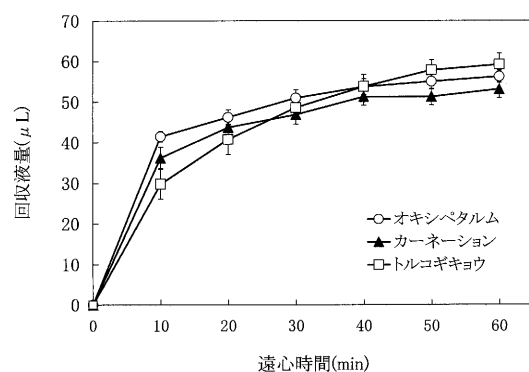
第5図 花弁の遠心時間と回収液量との関係 誤差線は標準誤差を示す
