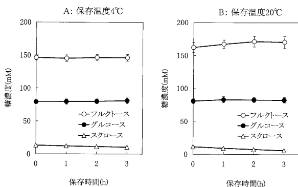
第3図 簡易迅速法で得られたパラ花卉抽出試料を異なる温度で保存した場合の時間経過による糖質組成の変化 誤差線は標準誤差を示す
