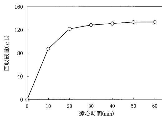
第 2 図 バラ花卉における遠心時間と回収液量との関係 誤差線は標準誤差を示す
