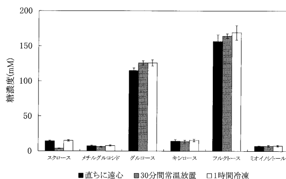
第4図 遠心前のパラ花卉の保存法と糖濃度との関係 誤差線は標準誤差を示す
