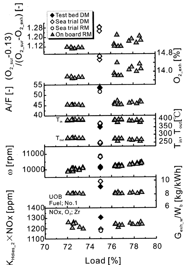
図-21 陸上、海上公試、運航中計測時の 計測及び算出項目の比較
