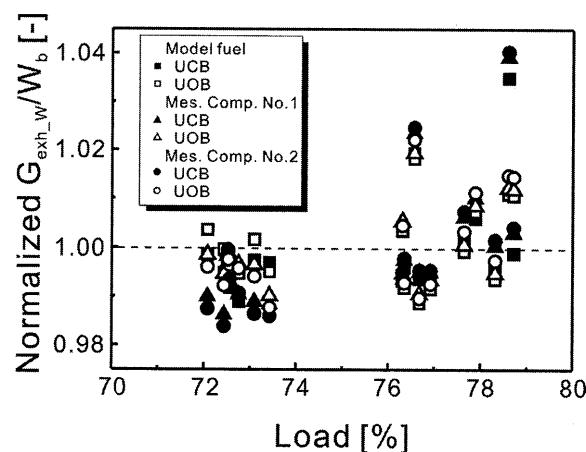
図-14 運航中での排ガス流量の差異
