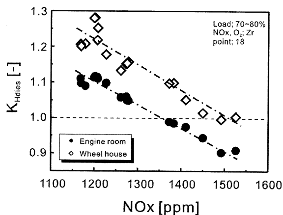
図-18 温湿度計測位置の排出濃度への影響
