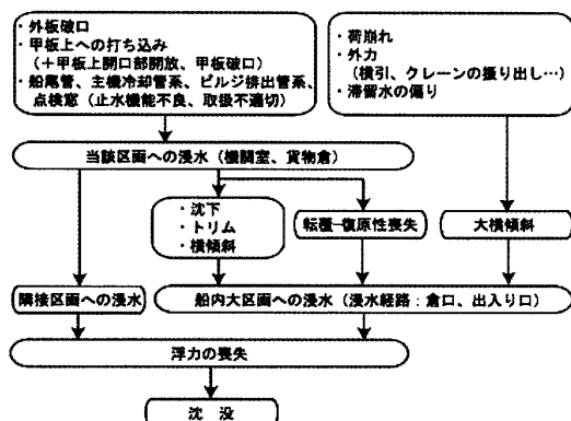
図 6 沈没事故シーケンスの類型化
