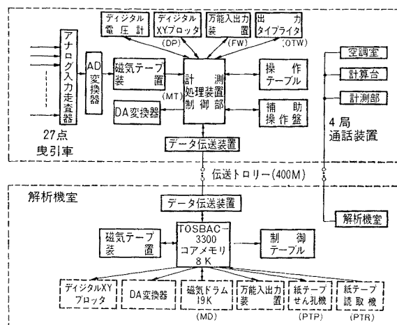
図3 水槽用解析設備の概要
