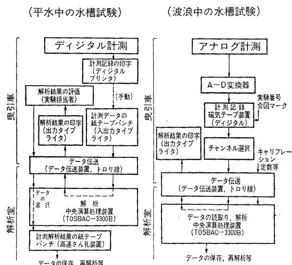
図1 船型試験水槽のオン・ライン・データ処理
