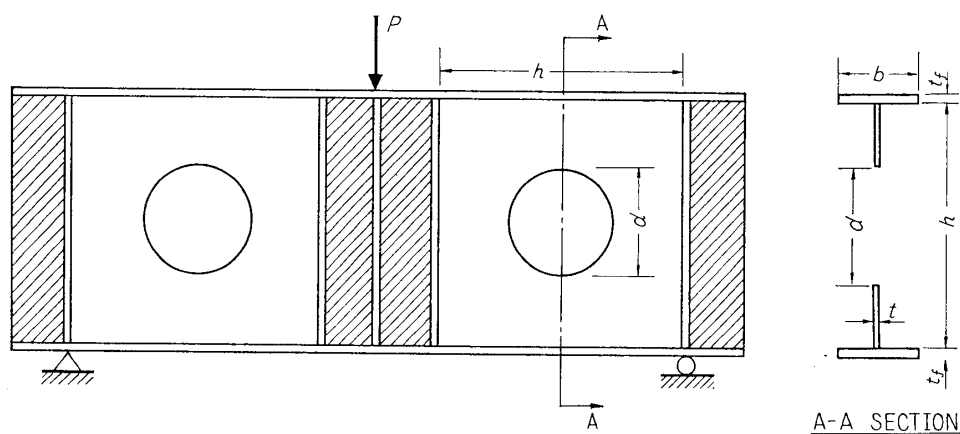
Fig. 7 Test setup
