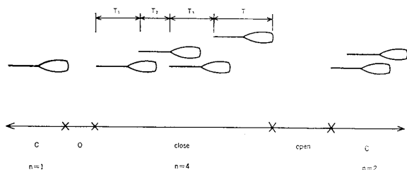
図-4 交差点の閉塞される時間間隔
