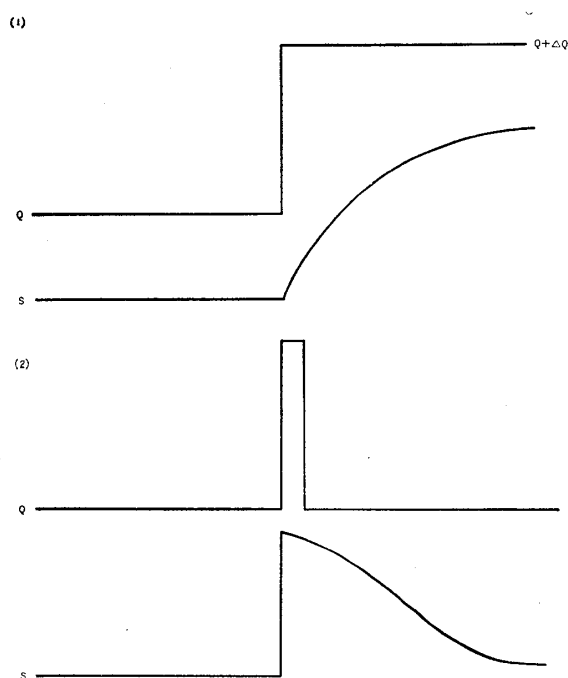
図-8 交通量が変化したときの待機隻数の変化
