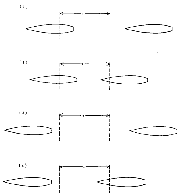
図-9 任意にとった時間間隔 \tau と、優先側船舶による閉塞時間との位相関係
