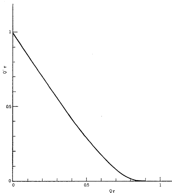
図-7 時間おくれ無限大となる時の Q' \tau と Q \tau の関係
