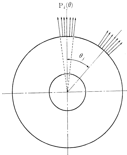
Fig. 3 外周上に discrete する荷重を受ける円板
