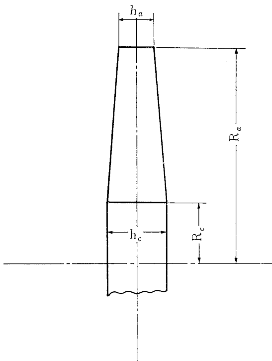
Fig. 4 厚さが直線的に変化する円板
