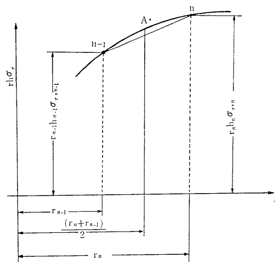
Fig. 5 n と (n-1) 点の間の中点の近似
