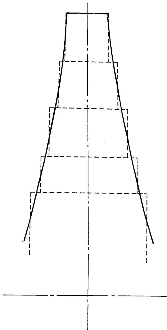
Fig. 1 任意の厚さを有する円板の分割
