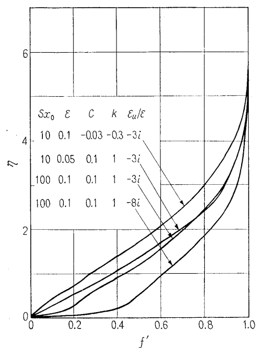
図-7 境界層内定常成分速度分布
