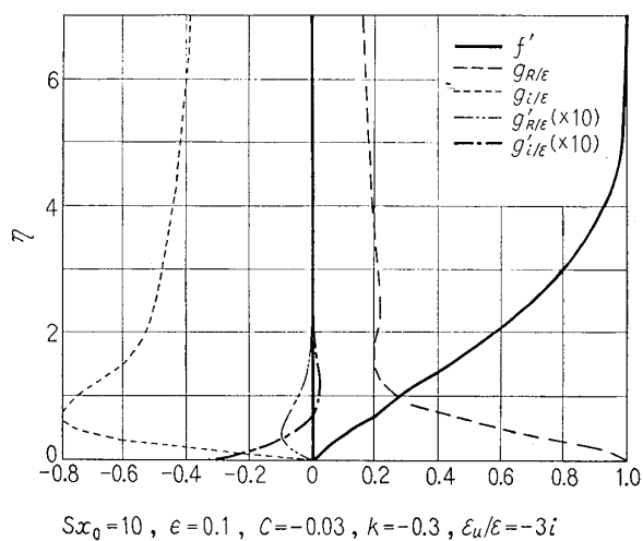
図-6 境界層内速度分布
