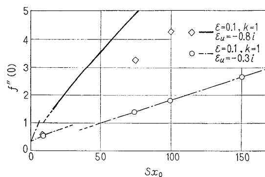
図-8 f''(0) の sx_0 に対する変化
