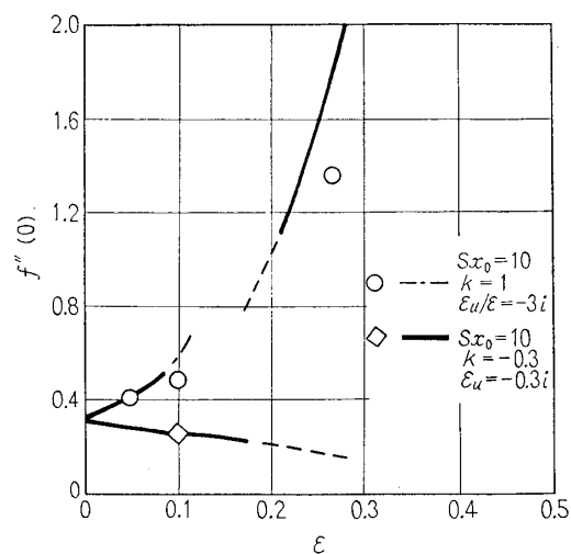
図-9 f''(0) の \epsilon に対する変化
