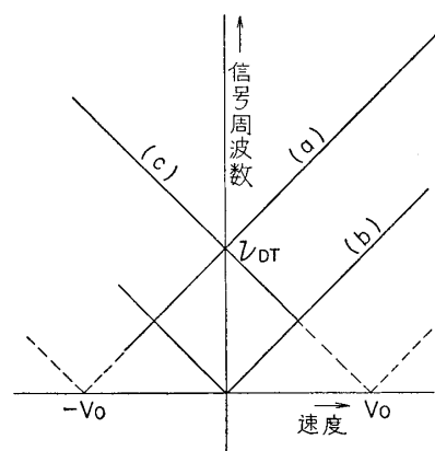
図-2.11 速度-信号周波数
