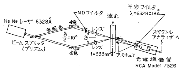
図-2.2 R.J. Goldstein らの光学系
