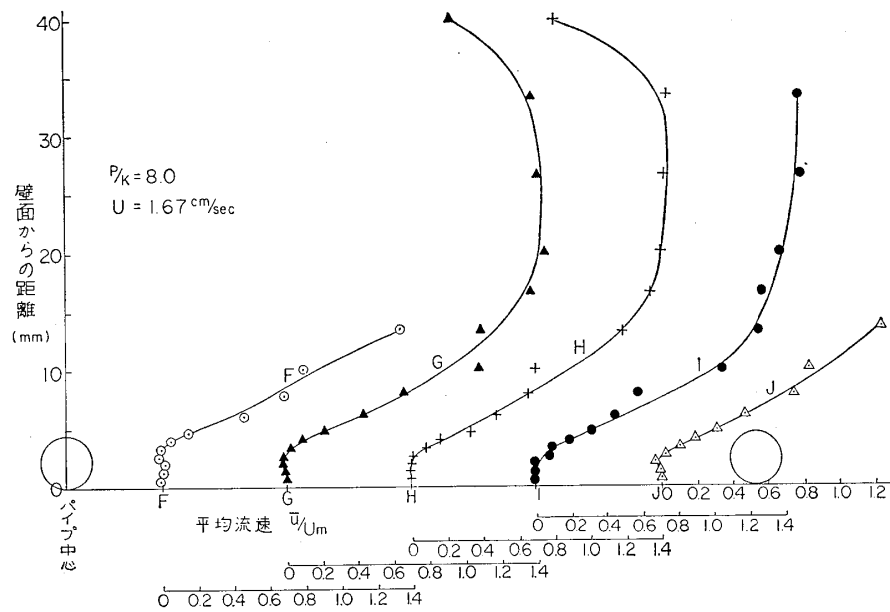
図-3-6 \bar{u}/U の Y 方向分布 ( P/k=8.00 , U=1.67 \text{ cm/sec} )
