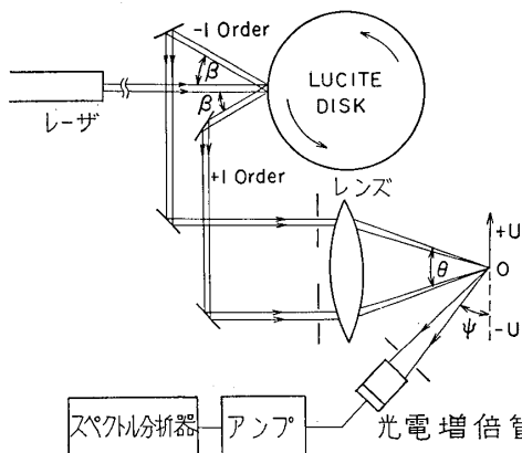
図-2.8 Mazumder による速度方向判別法
