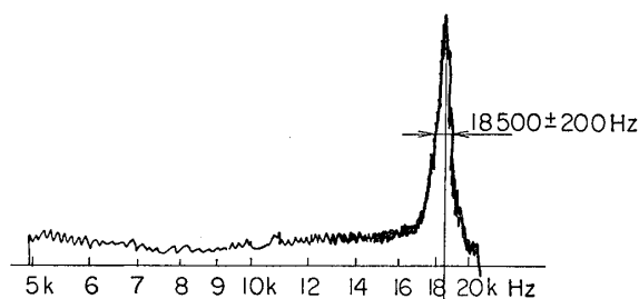
図-2.12 信号によるスペクトル
