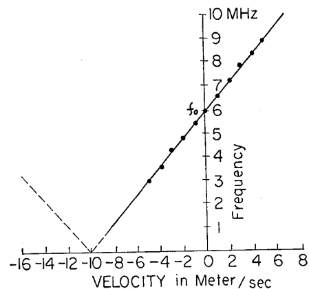
図-2.9 正負判別光学系による速度-信号周波数
