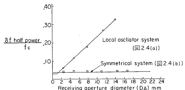
図-2.5 アパチュアの影響
