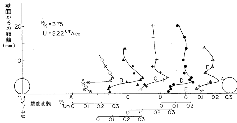
図-3-13 \bar{v}'/U の Y 方向分布 ( P/k=3.75 , U=2.22 \text{ cm/sec} )
