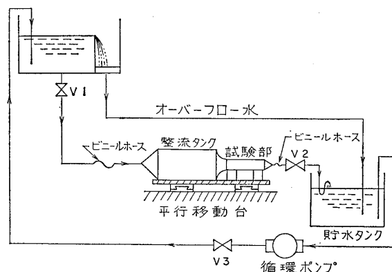
図-3.1 定流量装置
