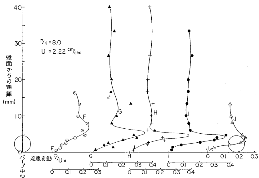
図-3-15 \bar{v}'/U の Y 方向分布 ( P/k=8.00 , U=2.22 cm/sec)
