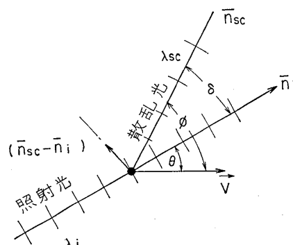
図-2.1 レーザドップラの原理
