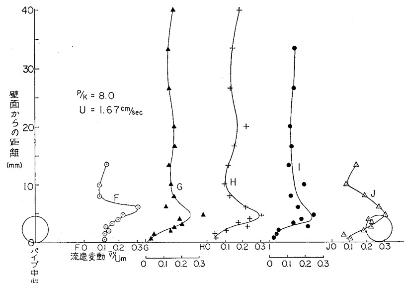
図-3-14 \bar{v}'/U の Y 方向分布 ( P/k=8.00 , U=1.67 \text{ cm/sec} )
