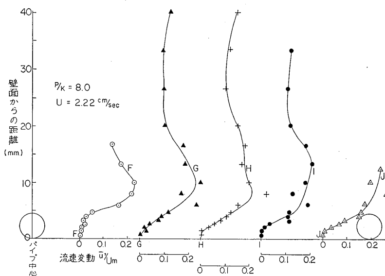
図-3-11 \bar{u}'/U の Y 方向分布 ( P/k=8.00 , U=2.22 cm/sec)
