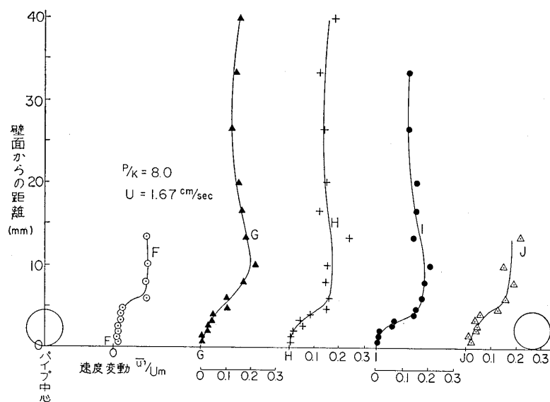
図-3-10 \bar{u}'/U の Y 方向分布 ( P/k=8.00 , U=1.67 cm/sec)
