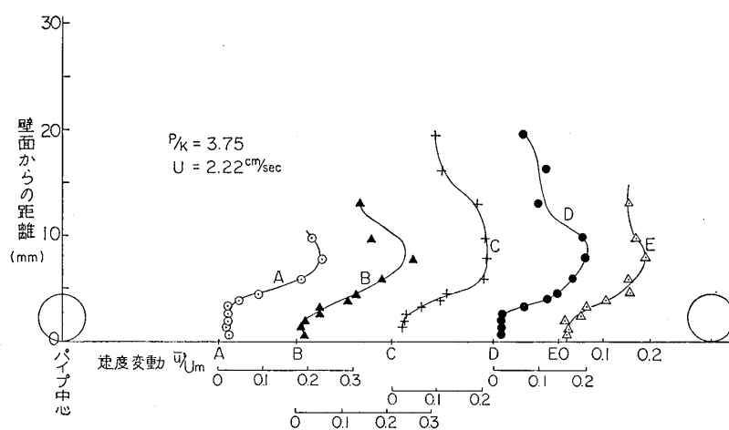
図-3-9 \bar{u}'/U の Y 方向分布 ( P/k=3.75 , U=2.22 cm/sec)
