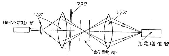
図-2.6 Rudd の方法
