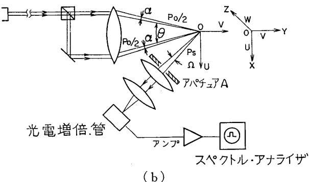
図-2.4 Mazumder, Wankum の方法
