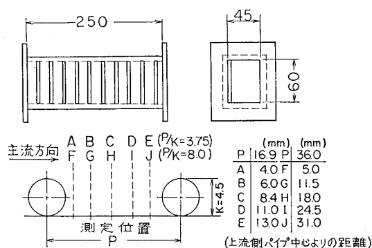
図-3.2 試験部
