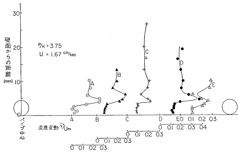
図-3-12 \bar{v}'/U の Y 方向分布 ( P/k=3.75 , U=1.67 \text{ cm/sec} )
