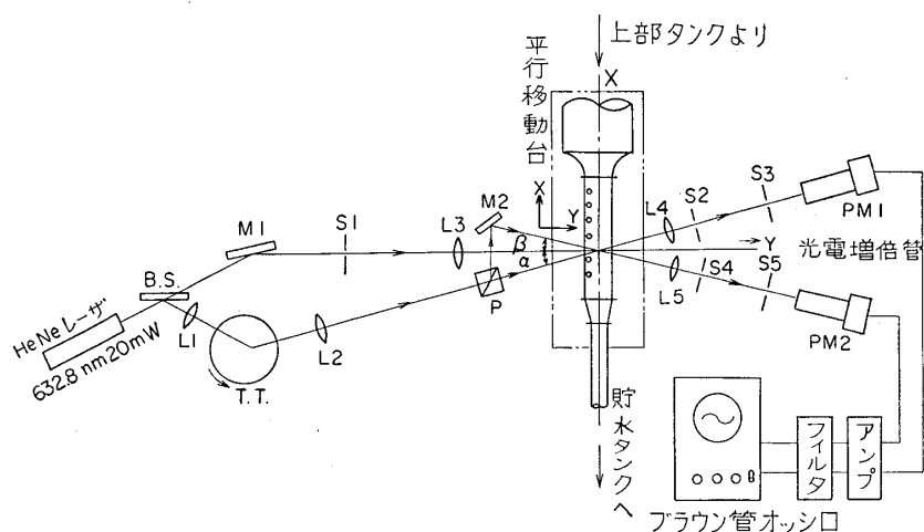
図-2.10 正負判別レーザー流速計
