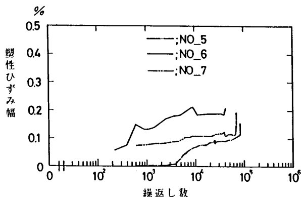
図3-12 塑性ひずみ幅と繰返し数の関係
