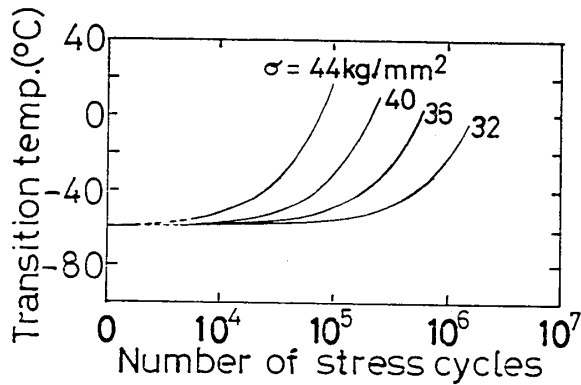
図4-1 S20C 鋼の片振引張疲労における繰返し応力、回数、および超音波遷移温度 11)
