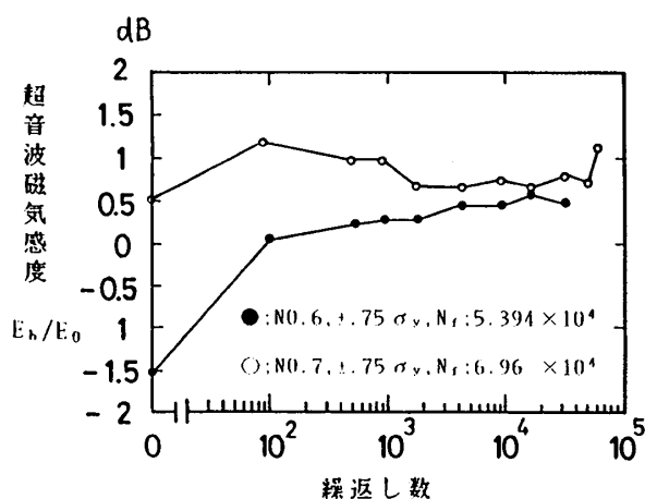
図3-13 永久ひずみを与えた場合の超音波磁気感度と繰返し数の関係
