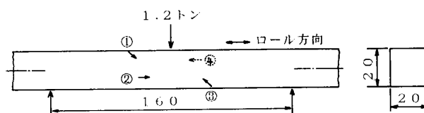
図3-1 3点曲げ疲労試験片, SM50 材(圧延材から加工), ○内数字は超音波測定面
