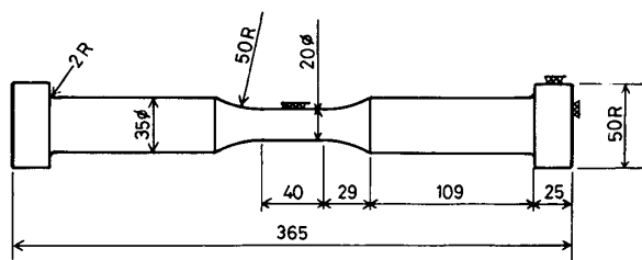
圖2-9 試驗片形狀
