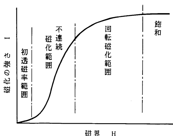
図2-12 磁化特性
