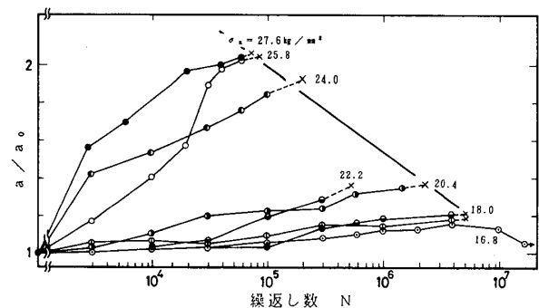
図2-7 a/a_0 と繰返し数との関係
