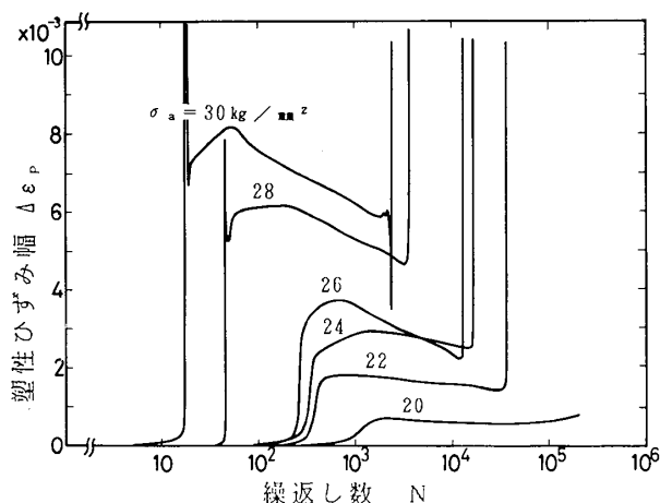
図2-16 疲労過程の塑性ひずみ幅
