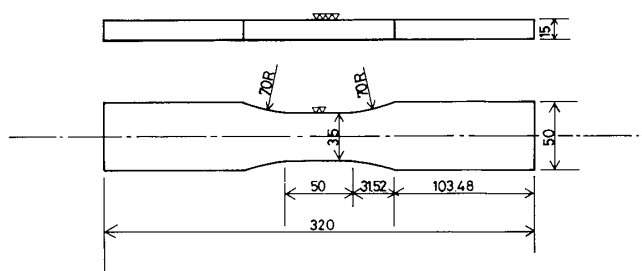
図2-24 試験片形状
