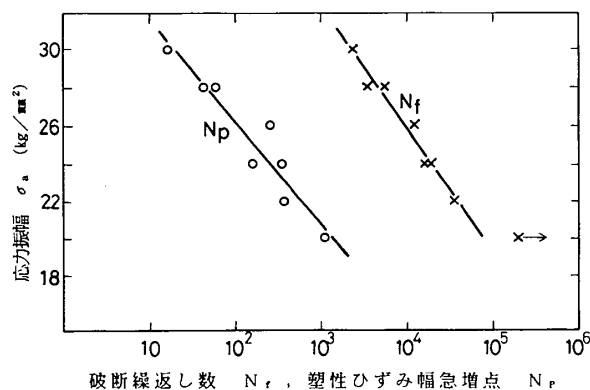
図2-17 各応力振幅における破断繰返し数と塑性ひずみ幅急増点
