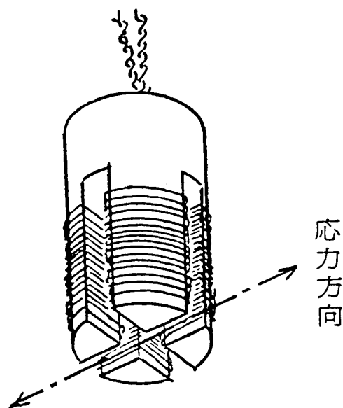
図2-26 磁気異方性センサ
