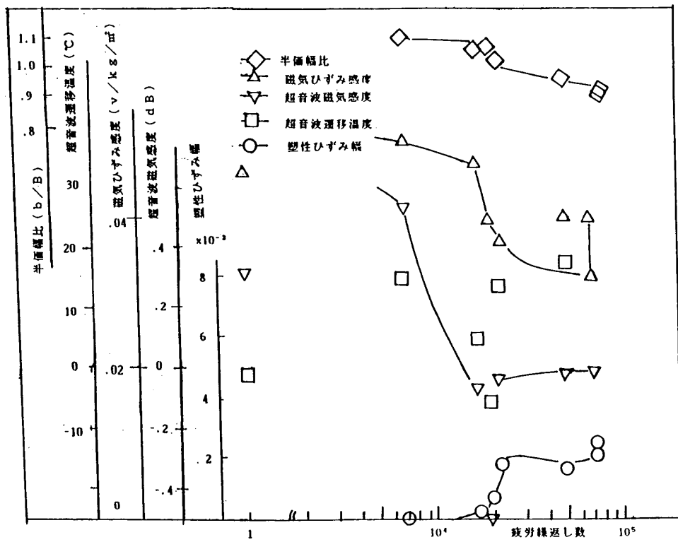
図5-1 応力振幅24kg/mm²における各計測法
