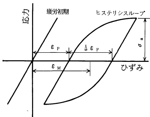
図2-15 応力-ひずみ線図
