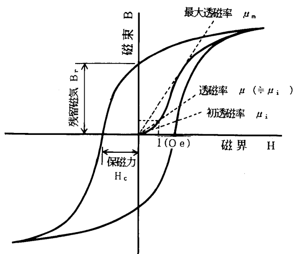
図2-13 磁気ヒステリシス曲線
