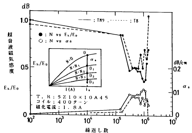
図3-5 シェンク疲労試験における繰返し数と超音波磁気感度の関係（試験片 TM 9, T 8）
