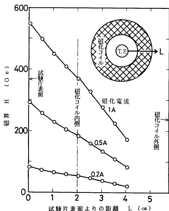
図2-11 試験片の外部磁界分布
