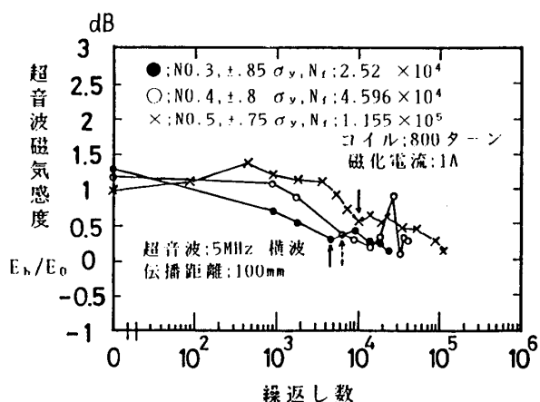
図3-11 超音波磁気感度と繰返し数の関係
