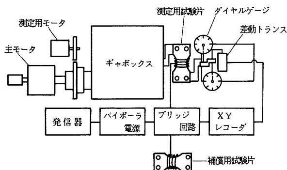
図2-2 試験装置概要
