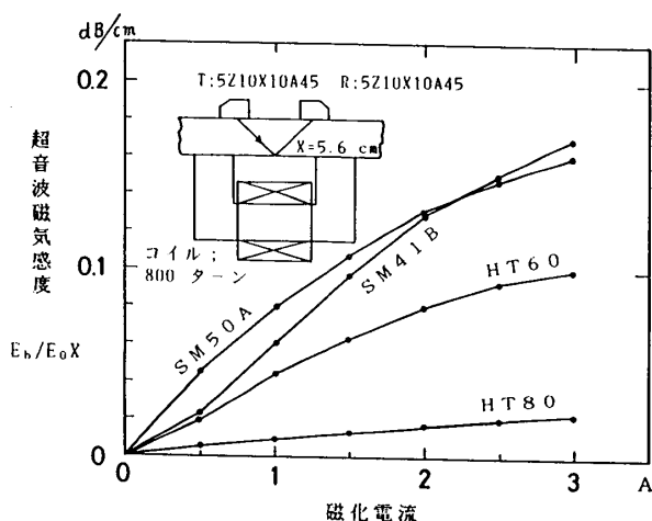
図3-14 構造用鋼における単位長さ当りの超音波磁気感度
