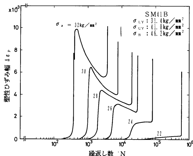
図2-27 疲労過程の塑性ひずみ幅
