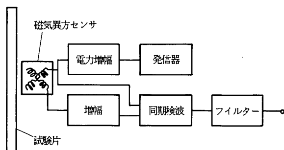
図2-25 磁気異方性センサ測定装置
