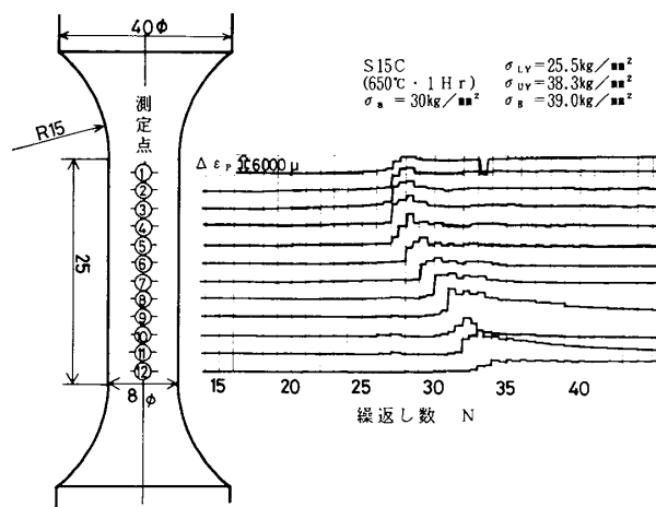
図2-18 試験片各点における塑性ひずみ幅挙動
