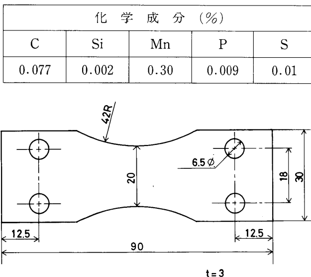
図2-1 試験片形状
