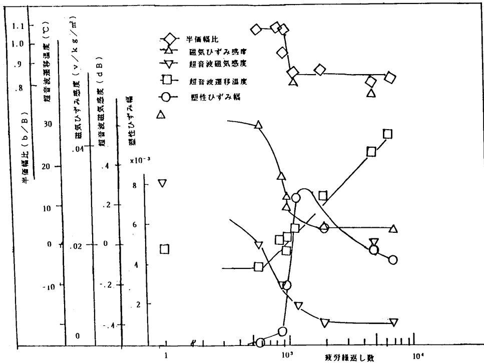
図5-2 応力振幅30kg/mm²における各計測法
