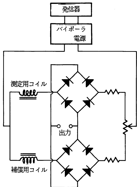
図2-4 ブリッジ回路
