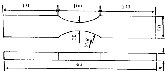
図3-10 試験片の形状および寸法
