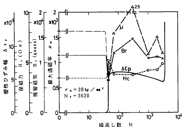
図2-20 疲労過程における磁気特性と塑性ひずみ幅
