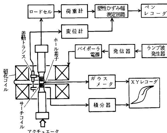
図2-10 試験装置概要
