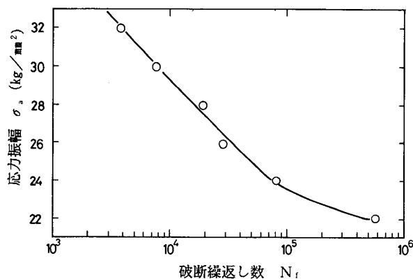
図2-28 S-N 線図
