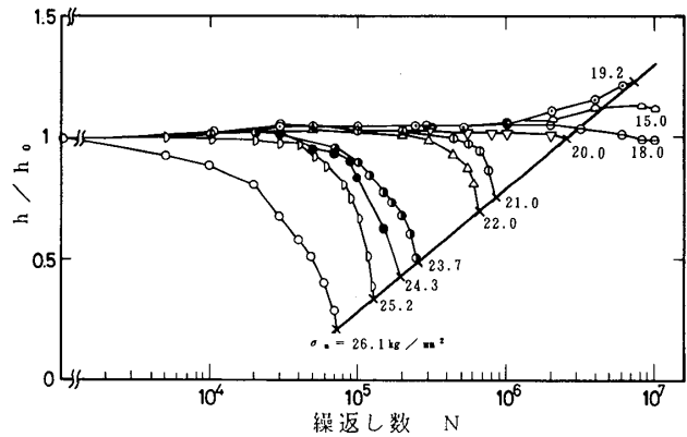
図2-6 h/h_0 と繰返し数との関係
