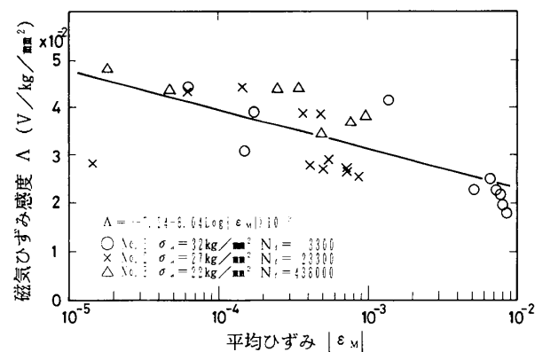
図2-32 磁気ひずみ感度と平均ひずみの関係
