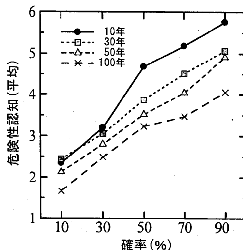
図2 期間ごとの危険性認知と確率の関係
