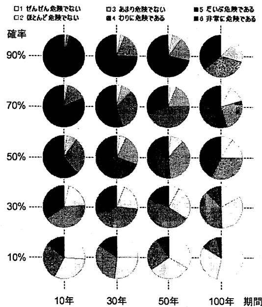
図1 期間・確率ごとの危険性認知
