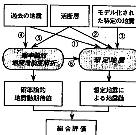
図-1 地震危険度評価のフロー
