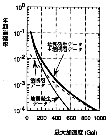
図-4 神戸におけるハザード曲線
