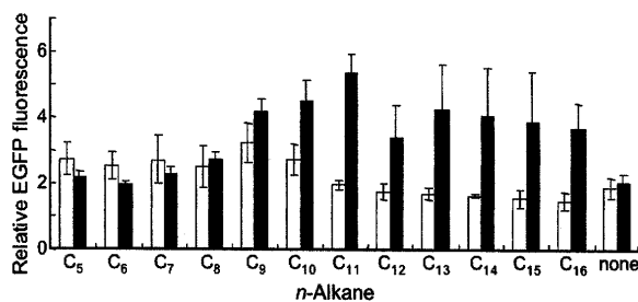
図1. 鎖長の異なる各種 n -アルカン添加24時間後の GFP 強度。水系（白）、有機溶媒系（黒）。
