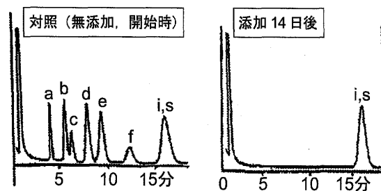
図7. 光合成細菌による低級脂肪酸の脱臭効果 3) 。ピーク：a, 酢酸；b, プロピオン酸；c, イソ酪酸；d, n -酪酸；e, イソ吉草酸；f, n -吉草酸；i, s, 標準マーカー。
