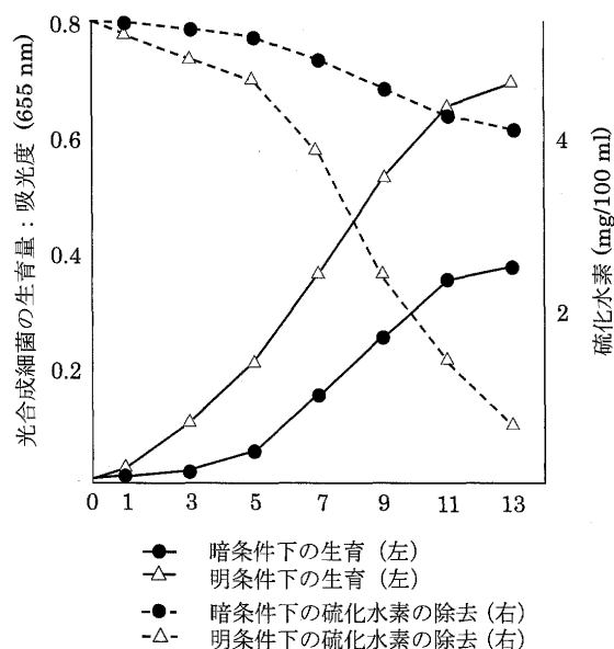
図1. 光合成細菌（ Chromatium sp.）の硫化ナトリウム培地中における生育と硫化水素の除去
