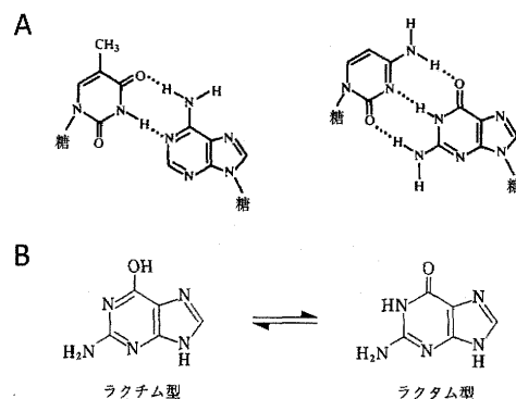
図1. DNAの塩基対形成と塩基の互変異性体。A, 中性付近での塩基対形成；B, グアニンのエノール型（ラクチム型）-ケト型（ラクタム型）互変異性体。
