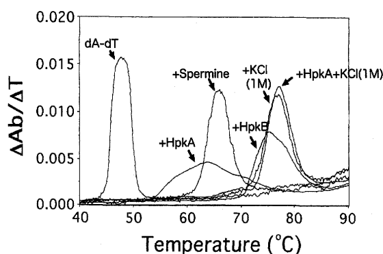
図2. DNAの T_m に及ぼすポリアミン、塩化カリウム、ヒストンの影響。poly (dA-dT) (10 \mu g) に対してスペルミン (10 \mu M)、塩化カリウム (1M)、二種類の超好熱菌ヒストンHpK A, HpK B (2.3 \mu M) を添加して融解温度に及ぼす影響を調べた。
