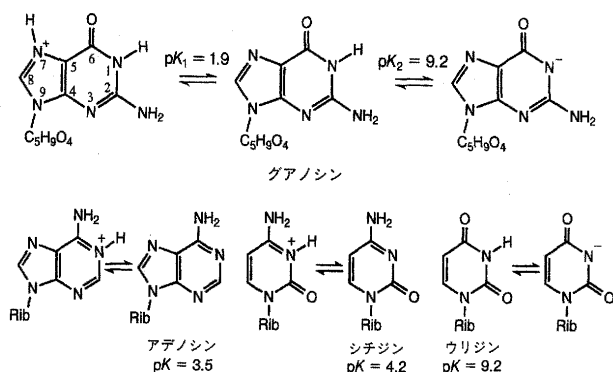
図4. 核酸構成塩基のイオン化. チミジンはウリジンと同様にイオン化する.
