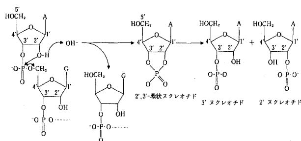
図5. 塩基触媒によるRNAの分解
