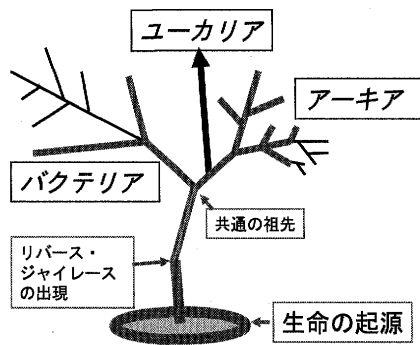
図6. 生物進化とリバーシジャイレースの出現時期. 図中の太い線は85°C以上で生育する超好熱菌を示す. リバーシジャイレースは, バクテリア, アーキアを問わずすべての超好熱菌に共通して存在することから, 共通祖先が分岐する前に誕生した可能性が高い.
