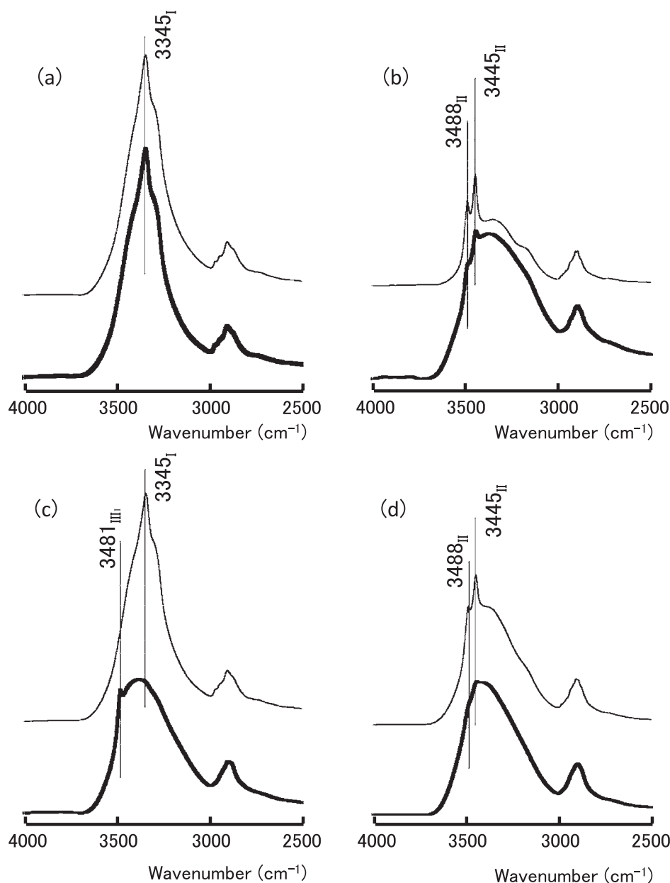
図4. セルロースの糖化前（太線）と糖化後（細線）の赤外吸収スペクトル. (a) セルロースI, (b) セルロースII, (c) セルロースIII, (d) リン酸膨潤セルロース.
