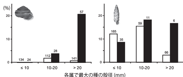
図7. カタツムリ (柄眼目) における、左巻きの種を含む属の割合。殻形態 (左: 平ら, 右: 細長), セダカヘビ科ヘビ類との分布重複の有無 (黒: 重複, 白: 無重複), および体サイズで区分して表示。グラフ上の数字は各カテゴリーに分類された属の総数。
