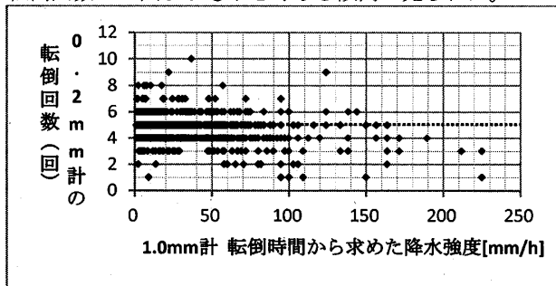
図 3 1.0mm 計で算出した降水強度と 0.2mm 計の転倒回数の関係（転倒回数 5 回、降水量 1.0mm を破線で示した）
