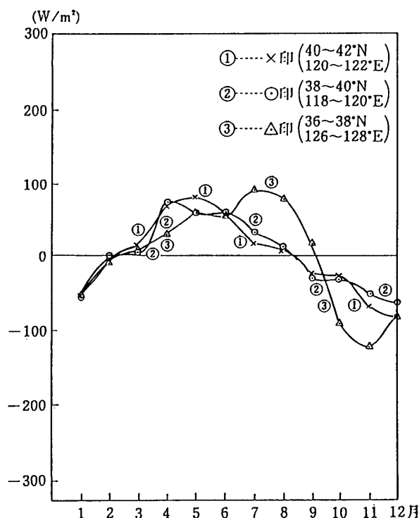
第7図 混合層相当の深さと表面水温を用いて求めた貯熱量 S ( \text{Wm}^{-2} ) の季節変化の例。 メッシュ① \times 印 ( 40\sim 42^\circ\text{N} , 120\sim 122^\circ\text{E} ) ② \circ 印 ( 38\sim 40^\circ\text{N} , 118\sim 120^\circ\text{E} ) ③ \triangle 印 ( 36\sim 38^\circ\text{N} , 126\sim 128^\circ\text{E} )
