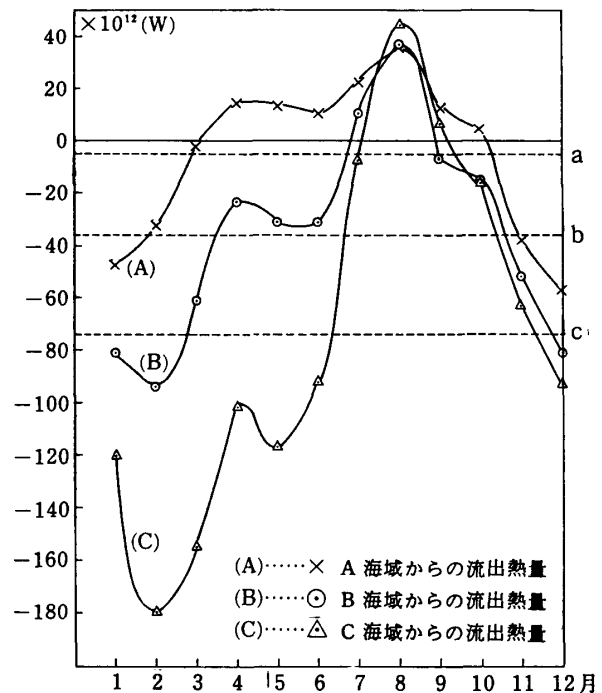
第11図 海洋運搬熱の発散量 F_{DIV} の面積分 F_T の季節変化
