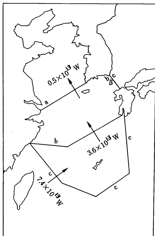
第13図 第12図に同じ，ただし年平均値。
