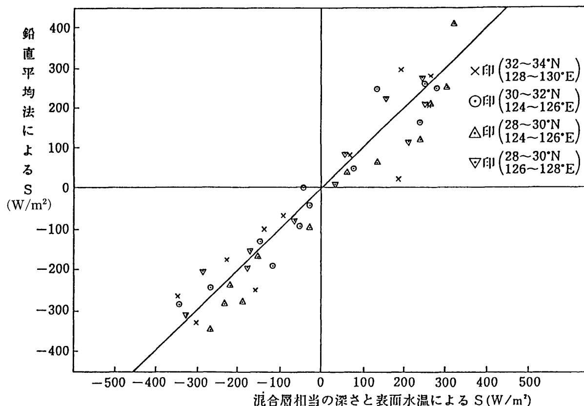
第6図 第5図と同じメッシュについて、「鉛直平均法」と「混合層相当の深さと表面水温による方法」の両方法で求めた S ( \text{Wm}^{-2} ) の比較.
