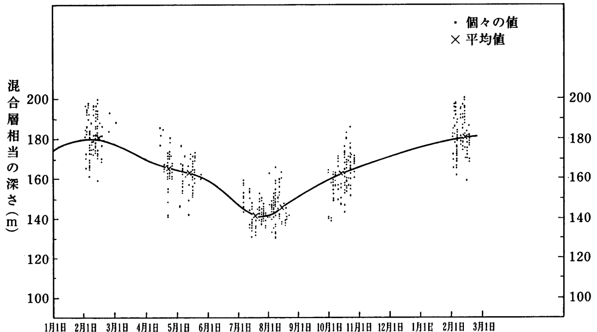
第3図 個々のデータによる混合層相当の深さ（ドット）と、それらの平均（×印）の季節変化の例。メッシュ（30~32°N, 128~130°E）。
