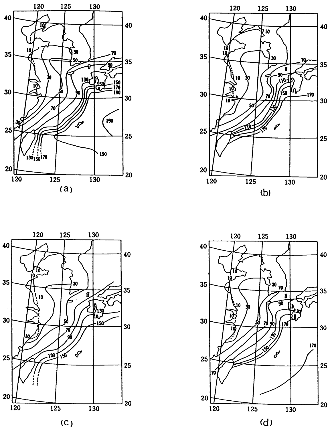
第4図 混合層相当の深さ1 (m)の分布図。1を推定したメッシュは、破線で描いてある。(a) 2月, (b) 5月, (c) 8月, (d) 11月.
