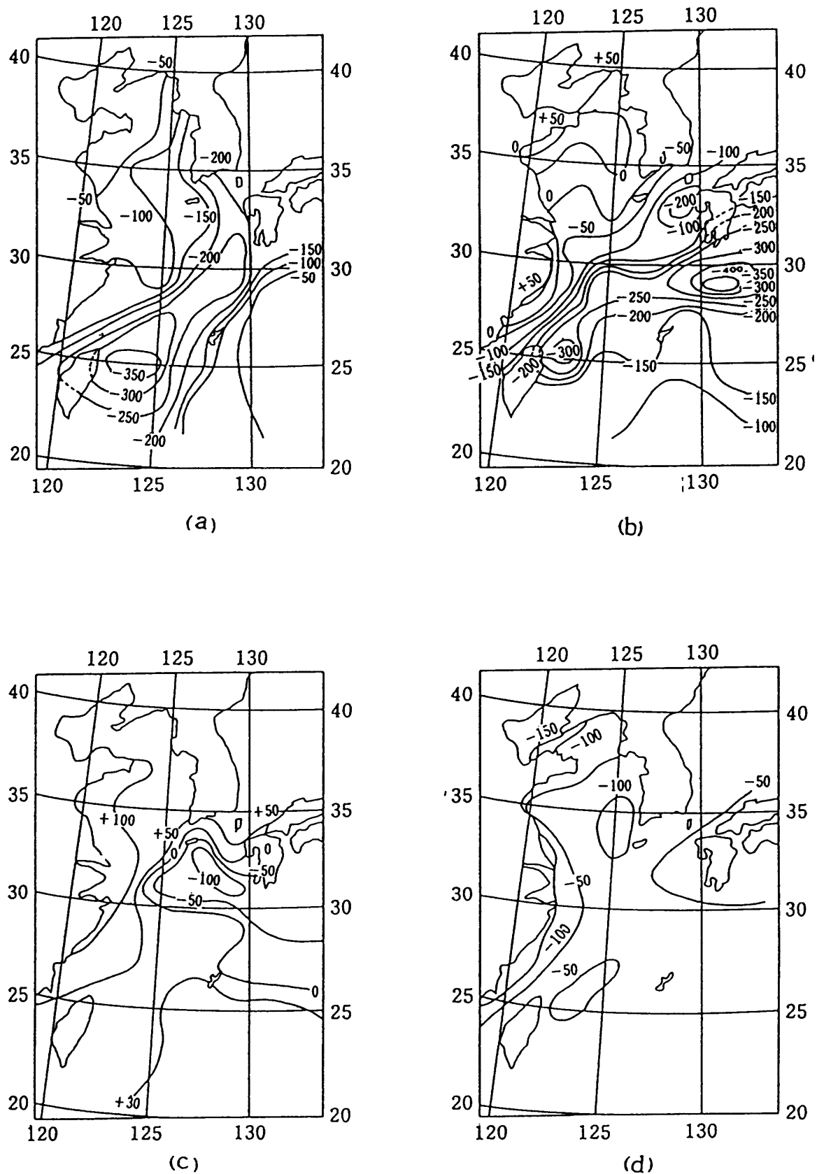
第9図 海洋運搬熱の発散量 F_{DIV} ( Wm^{-2} ) の分布. (a) 2月, (b) 5月, (c) 8月, (d) 11月.
