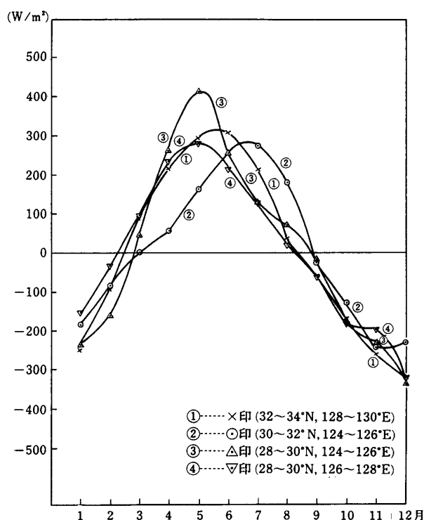
第5図 貯熱量 S ( \text{Wm}^{-2} ) を鉛直方向の平均水温を使って求めた例。
