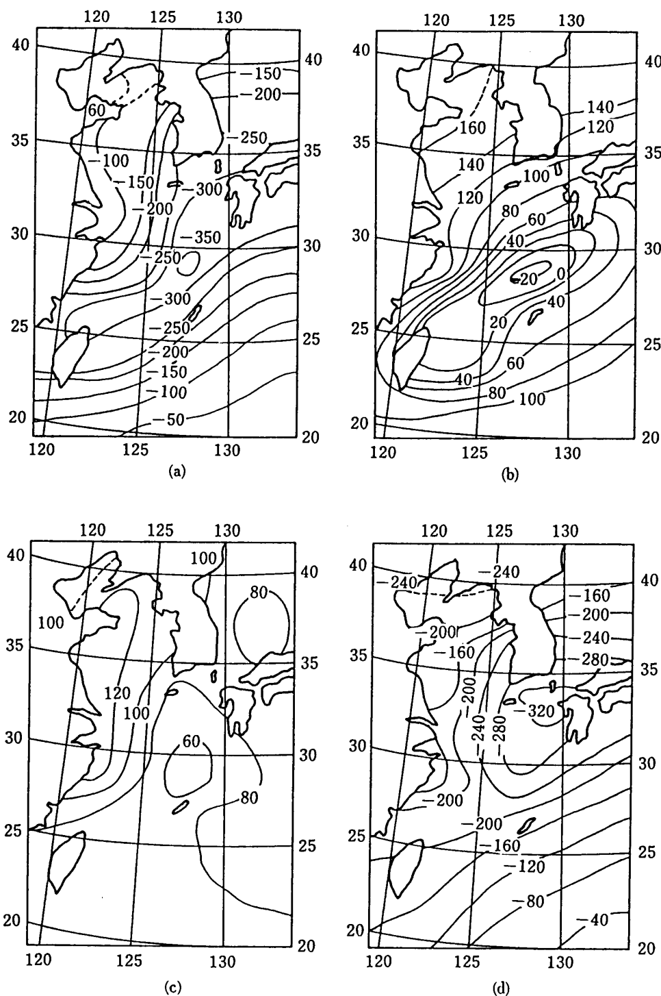
第10図 大気から海への正味の熱フラックス G ( \text{Wm}^{-2} ) の分布, (a) 2月, (b) 5月, (c) 8月, (d) 11月, (石井・近藤, 1987より再掲). ただし前報告における Q は本論文では記号を替え G としてある.
