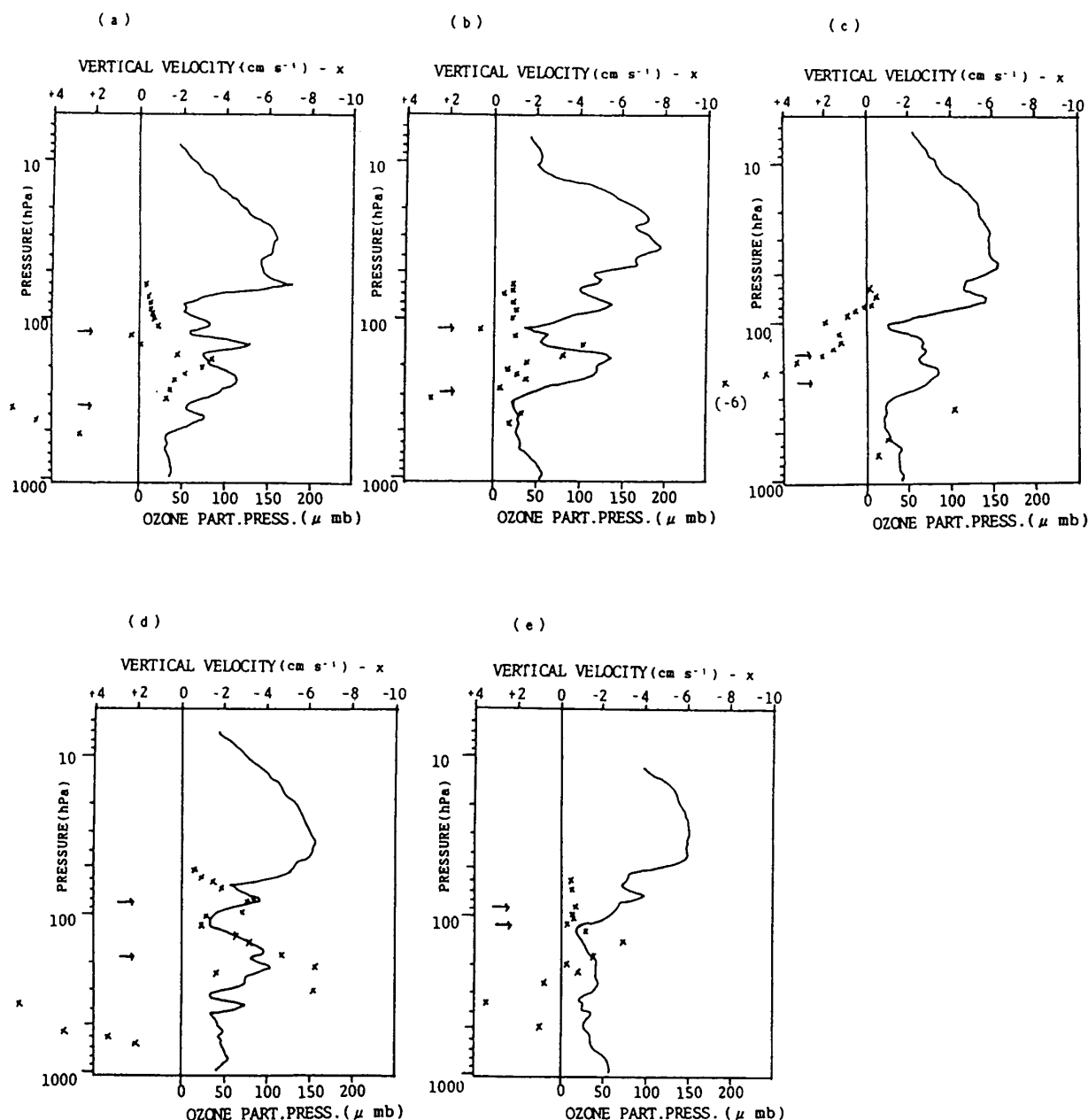
第2図 エアロロジカルデータオゾン特別号からの1986年3月20日(a), 3月26日(b), 4月23日(c), 5月16日(d), 5月28日(e)の各14時30分(JST)頃についてのオゾン鉛直分布( \mu\text{mb} )と鉛直流( \text{cm s}^{-1} , 正が上昇)との関係。矢印は第一圏界面及び第二圏界面を示す。
