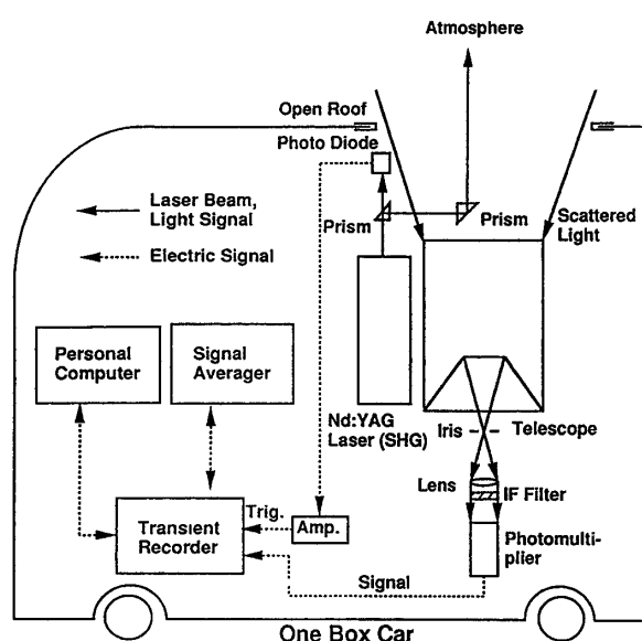
第4図 車載型ミ一散乱ライダーシステム
