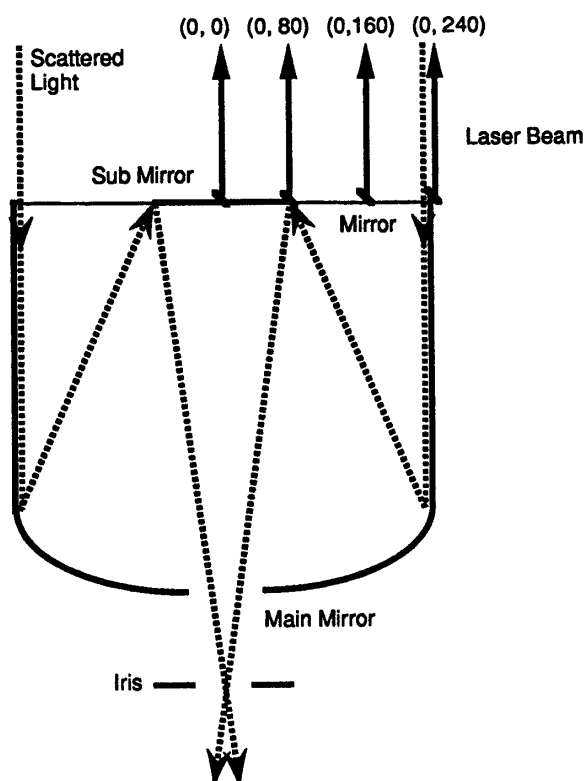
第1図 送受信光学系配置図.
