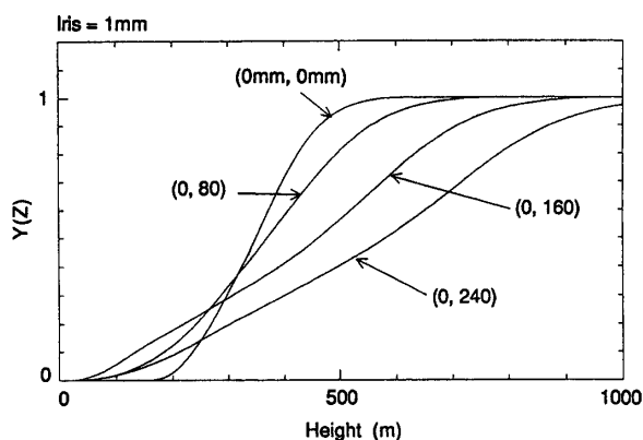
第2図 視野重なり関数の計算結果例.
