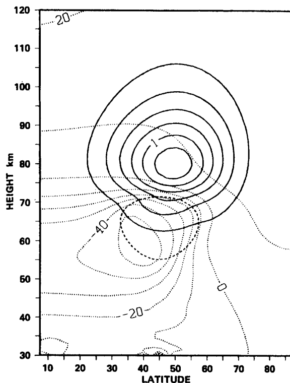
第7図 第6図の場合における最大成長率を持つ不安定波動の振幅 (実線, 単位は任意) と位相 (点線, 単位は度). 東西波数 = 3. Pfister (1985) より引用.
