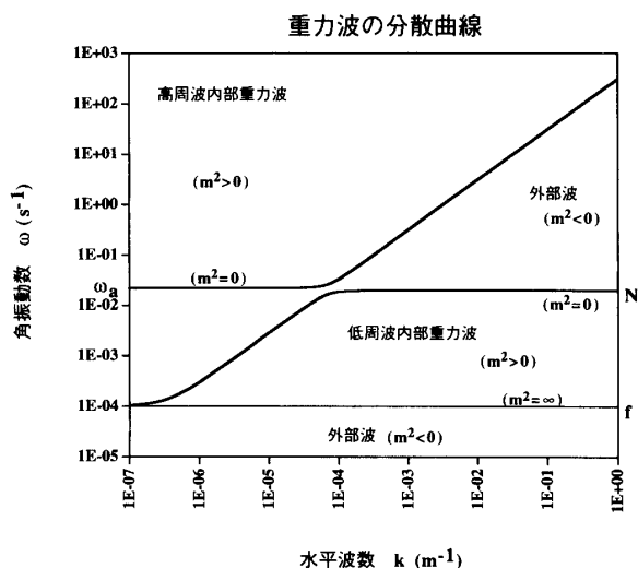
第 1 図 重力波の分散関係。振動数の大きい高周波内部重力波（浮力により変形された音波）と小さい低周波内部重力波（浮力を復元力とする波）の 2 種類の波動が存在する。
