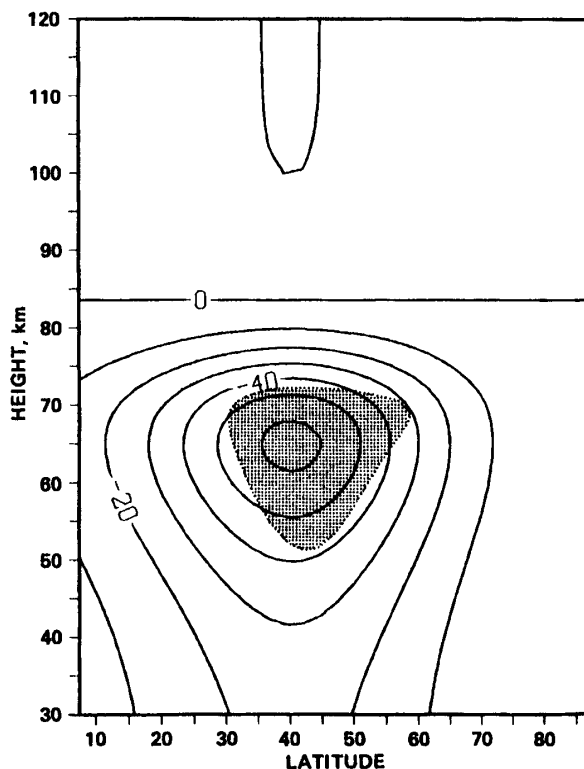
第6図 夏の模式的東風ジェット分布. 単位は \text{ms}^{-1} . 陰影部分は \overline{q_y} が負となる部分を示す. Pfister (1985) より引用.
