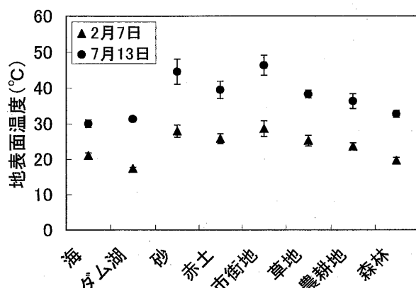
第3図 2月7日(冬季)と7月13日(夏季)の土地被覆ごとの地表面温度観測値。プロットは平均値、縦の線は平均値からのばらつきの標準偏差。いずれも直達日射が雲で遮られなかった画像のみを対象(冬季23画像、夏季67画像)。
