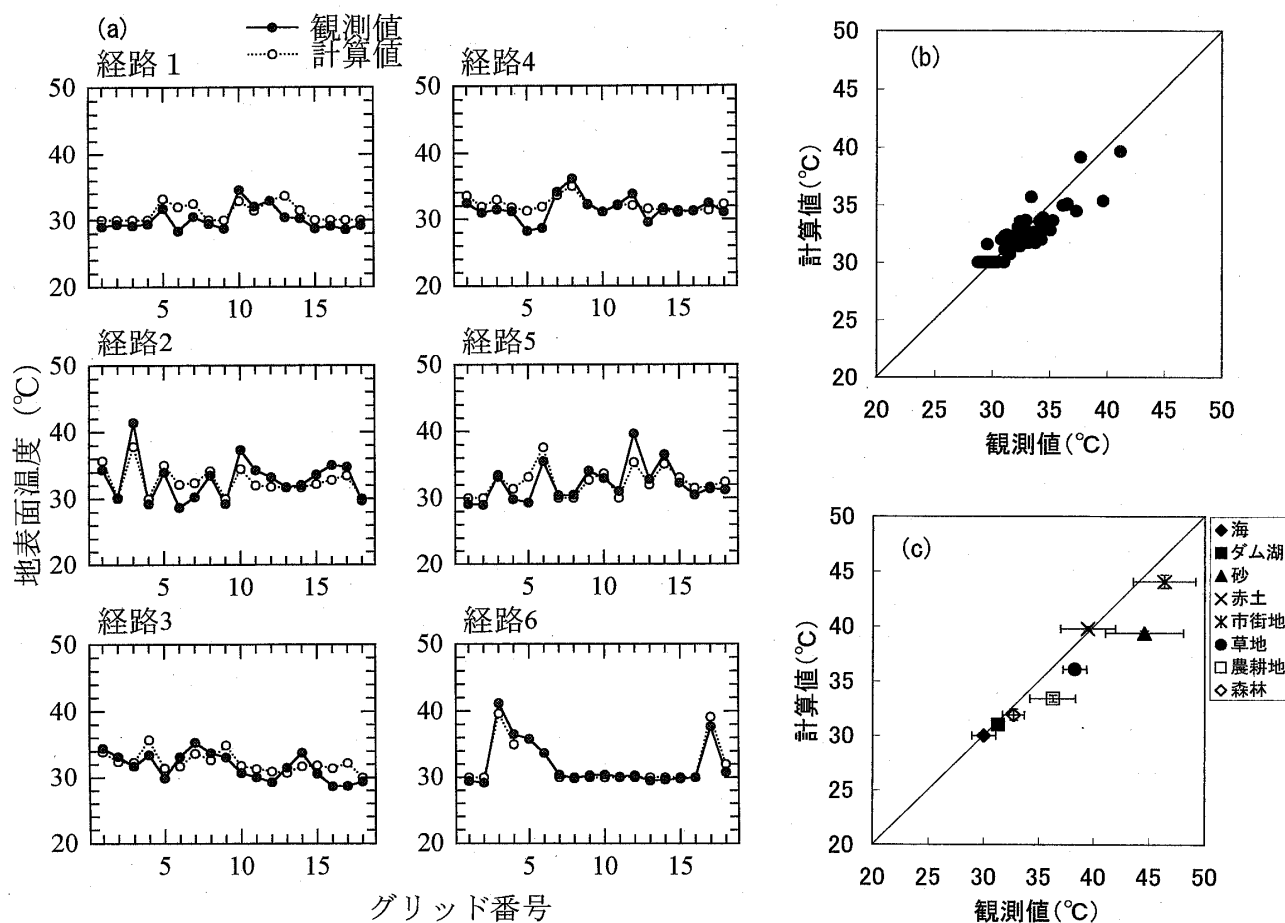
第5図 第4図と同じ。ただし、7月13日。
