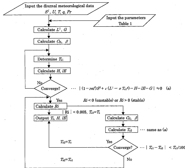
第2図 熱収支計算の流れ図.
