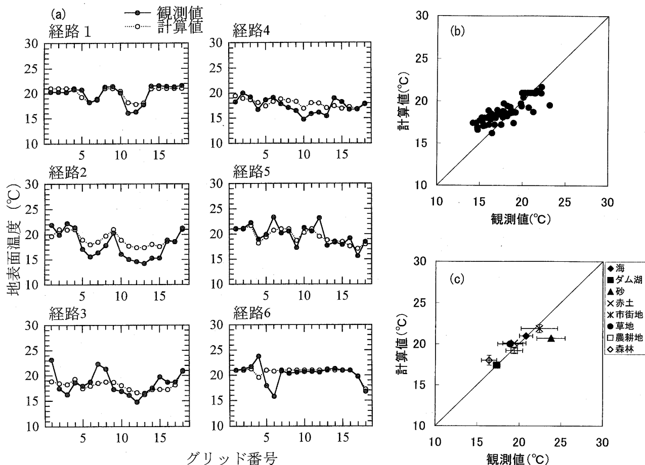
第4図 2月7日における地表面温度の観測値と計算値の比較。(a) 各経路における観測値と計算値の比較。横軸は各経路のグリッド番号、縦軸は地表面温度。(b) (a)を散布図にしたもの。(c) 土地被覆別の観測値と計算値の比較。プロットは平均値、縦の線、横の線はそれぞれ計算値および観測値の平均値からのばらつきの標準偏差。
