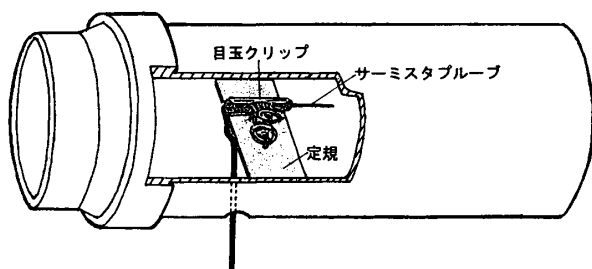
第2図 Radiation shield.
