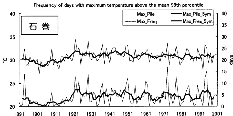
第3図 石巻における「暑い日」の経年変化 (中三川, 2002). 上段は各年で4番目に高い日最高気温, 下段は各年の「暑い日」. 太線は5年移動平均. 各年の高いほうから4番目 (365日の上位1%の値) の日最高気温を1961～1990年の30年間で平均した値を求め, この値を上回る日数を「暑い日」と定義.
