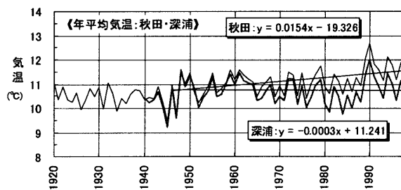
第2図 秋田 (1920～1997年), 深浦 (1940～1997年) の年平均気温の経年変化 (竹川, 1999). 細線 (黒) は秋田, 太線 (灰色) は深浦. 図中の直線は1946～1997年のトレンド直線, 数式は直線を表し X の係数がトレンド量 (°C/年). 縦軸は年平均気温 (単位°C), 横軸は経過年.
