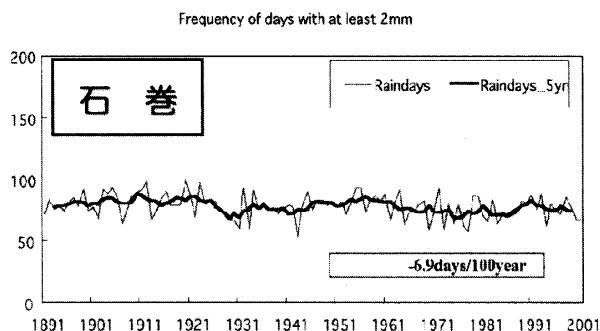
第7図 石巻における「降水日数」経年変化(中三川, 2002)。「降水日数」: 日降水量2mm以上の年間日数。太線は5年移動平均。
