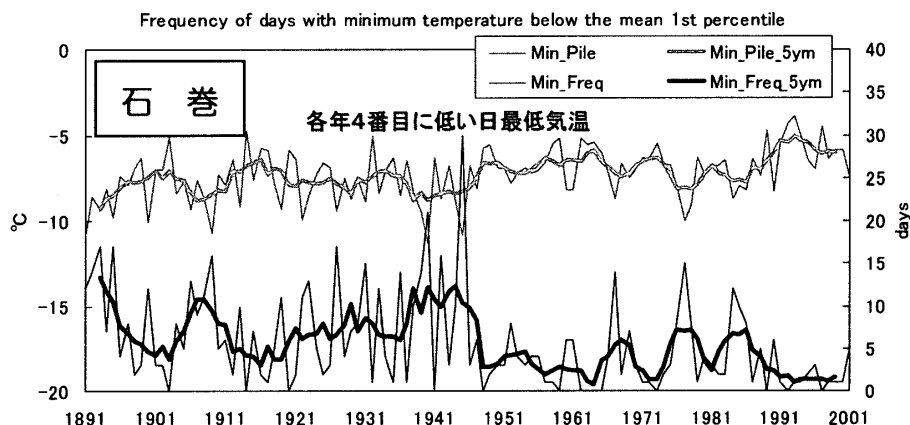
第4図 第3図と同様, ただし「寒い夜」の統計 (中三川, 2002). 上段は各年で4番目に低い日最低気温, 下段は各年の「寒い夜」. 各年の低いほうから4番目 (365日の下位1%の値) の日最低気温を1961～1990年の30年間で平均した値を求め, この値を下回る日数を「寒い夜」と定義.
