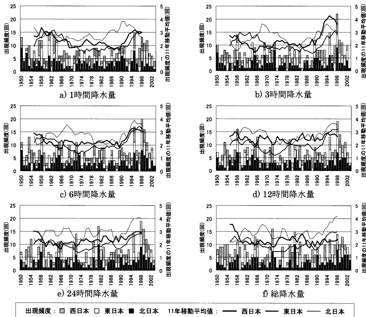
第5図 暖候季における再現期間が2年以上の大雨の出現頻度の時系列と11年移動平均値（地域別）。
