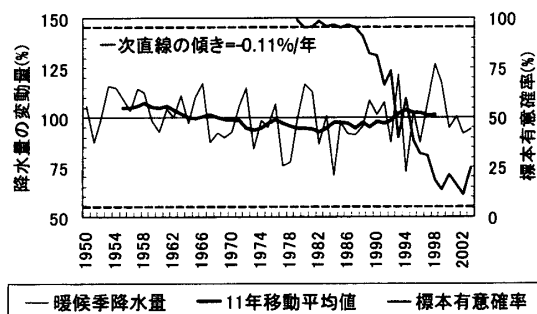
第4図 規格化した暖候季降水量の時系列, 11年移動平均値, 及び前30年間に「上昇傾向がある」に対する標本有意確率。
