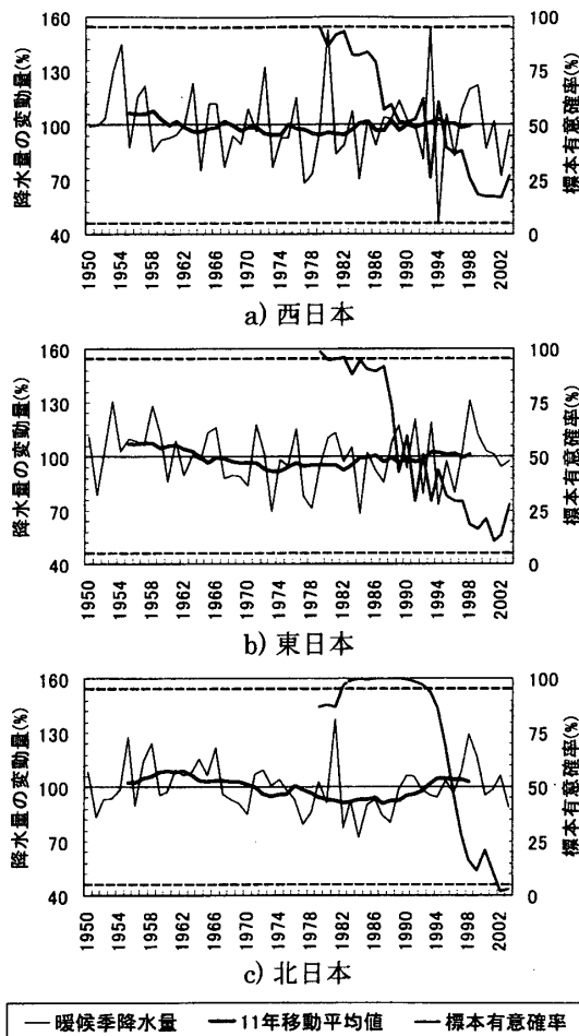
第7図 規格化した暖候季降水量の時系列, 11年移動平均値, 及び前30年間に「上昇傾向がある」に対する標本有意確率(地域別)。
