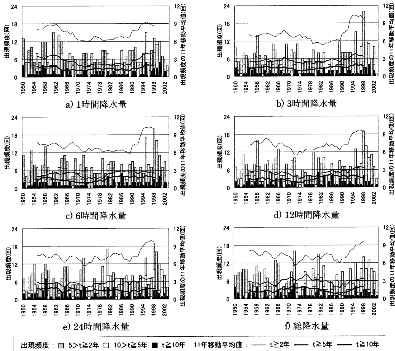
第2図 暖候季における大雨の出現頻度の時系列と11年移動平均値。
