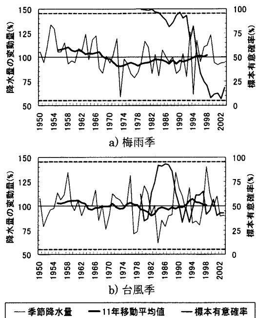
第10図 規格化した季節降水量の時系列, 11年移動平均値, 及び前30年間に「上昇傾向がある」に対する標本有意確率（全国）.
