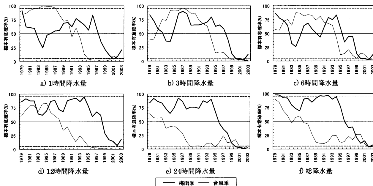
第9図 梅雨季と台風季における再現期間2年以上の大雨の出現頻度の前30年間に「上昇傾向がある」に対する標本有意確率（全国）.
