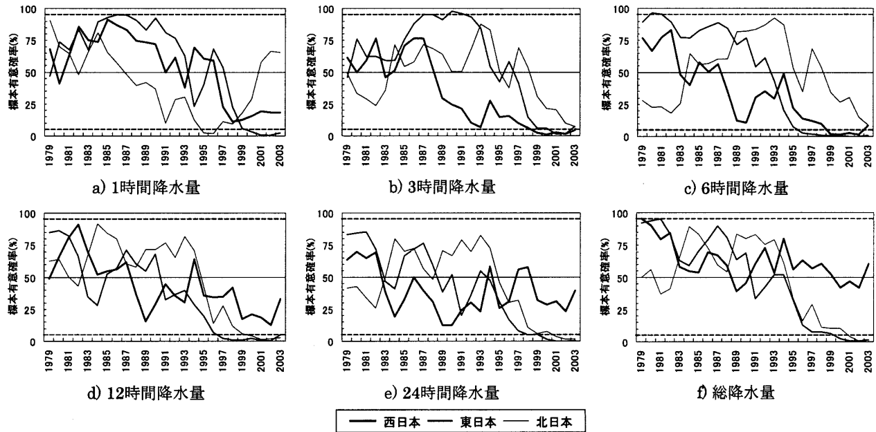
第6図 暖候季における再現期間が2年以上の大雨の出現頻度の前30年間に「上昇傾向がある」に対する標本有意確率(地域別)。
